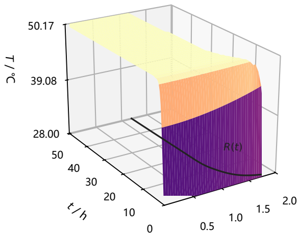
(b) 温度场 T(r, t) : 热场准稳态
