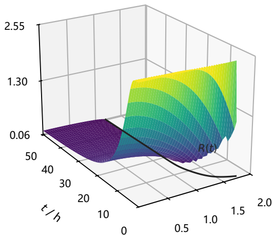
(a) 水分场 C(r, t) : 锋面内移
