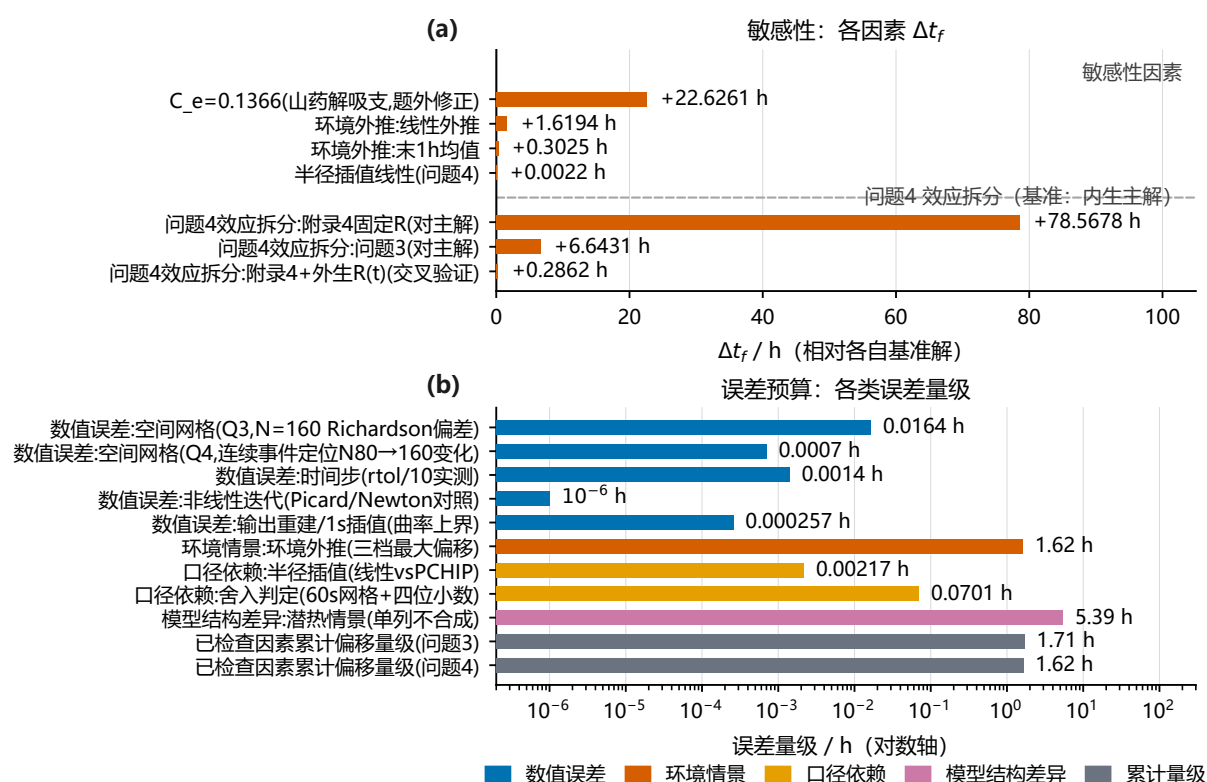
图 17 敏感性条形图(回答“结论有多稳”): 各因素 \Delta t_f 横向条形——边界汇口径 C_e = 0.1366 (题外修正) +22.63 h 自然主导, 环境外推 +1.62 h 次之, 半径插值仅 +0.002 h; 诚实展示最大不确定性来源, 主结果一律用声明闭合口径。
