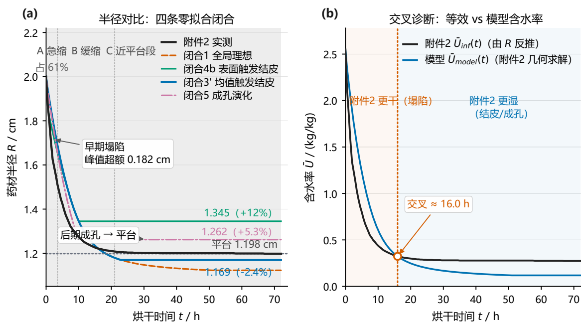
图 8 收缩机制分析（回答“附件 2 是什么样的收缩”）：附件 2 三段复合结构（A 急缩 61%/B 缓缩/C 平台）与约 16 h 滞后交叉；零拟合的“理想收缩 + 玻璃化冻结”半经验闭合已能结构性给出减速与平台（均值触发那一条：平台 1.169 cm、偏差 -2.4%、冻结时刻偏差 +12%），早期塌陷与后期成孔对应两组机制。数据源：附件 2 与问题 4 主解湿度场。
