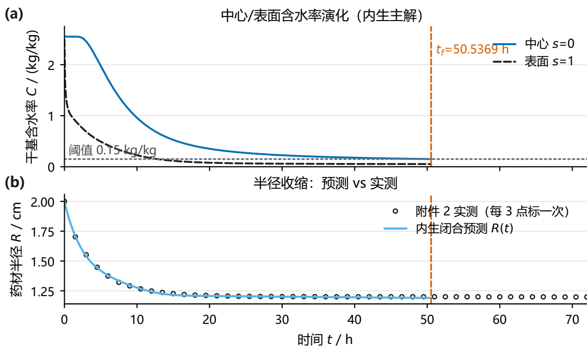
图 10 中心/表面含水率演化与半径收缩 (回答“达标过程如何推进”): (a) 中心与表面含水率曲线 + 0.15 kg/kg 阈值虚线 + t_f = 50.5369 h 达标竖线——表面先到干态、中心最后达标; (b) 内生半径 R(t) : 50.5 h 进入近平台, 60–72 h 仅再降 0.31 mm。
