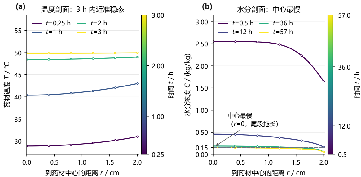
图 6 温湿剖面演化 (回答”场长什么样”): 代表时刻的径向温度/水分浓度剖面 (viridis 时间色阶)——表面先干、中心最慢、尾段拖长。
