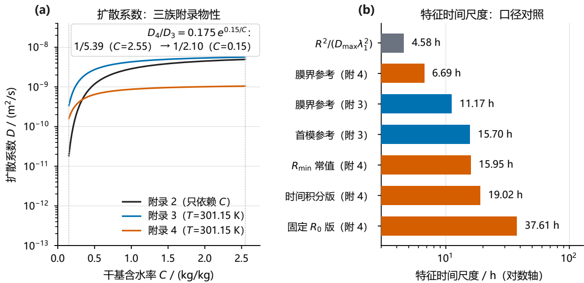
图 2 扩散系数非线性与特征时间尺度（回答”为什么难、量级多少”）：(a) 附录 3/4 的 D(C, T) 半对数曲线——尾段 ( C \rightarrow 0.15 ) D 缩小 16.8 倍，附录 4 全程低于附录 3；(b) 各参考时标：常系数首模参考 15.7021 h、膜界 11.1720 h、问题 4 瞬时首模时间积分 19.016 h、固定 R_0 版 37.61 h、 R_{\min} 常值版 15.95 h——主值 57.18/50.54 h 均远大于各时标。
