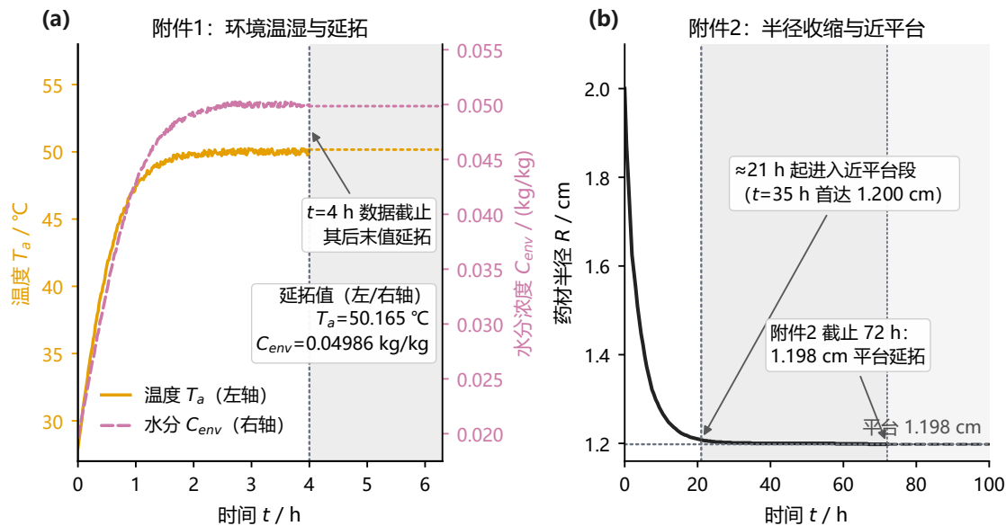
图 3 输入数据（回答”数据可用性如何裁定”）：附件 1 烘房温度与空气水分浓度（0–4 h、60 s 步）及末值保持外推；附件 2 外半径（0–72 h）的三段结构（急缩/缓缩/平台）与约 21 h 的近平台起点。
