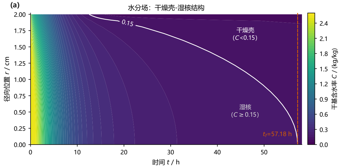
图 7 水分场时空演化（回答“干壳/湿核如何形成”）：时间 \times 径向位置的水分浓度云图——干燥锋面内移、表面快速进入低 D 区形成干壳，中心湿核维持到 40 h 以后；等值线给出 0.15 kg/kg 达标线，中心最后穿越。
