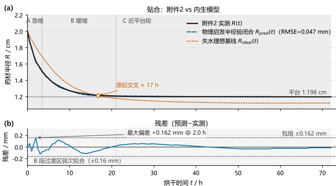
图 9 内生收缩模型对附件 2 的贴合与验证（回答“收缩能否由模型内生预测”）：三项物理动机机制的半经验闭合（式 (5.4)，5 个标定参数 + 2 个非拟合量）复现附件 2——RMSE 0.047 mm（量化分辨率的 5 倍）、滞后交叉（17.0 h vs 约 16 h）、平台（1.1969 vs 1.198 cm）、三段形态全对；残差子图显示偏差有界在 \pm 0.16 mm（单向拟合口径）。
