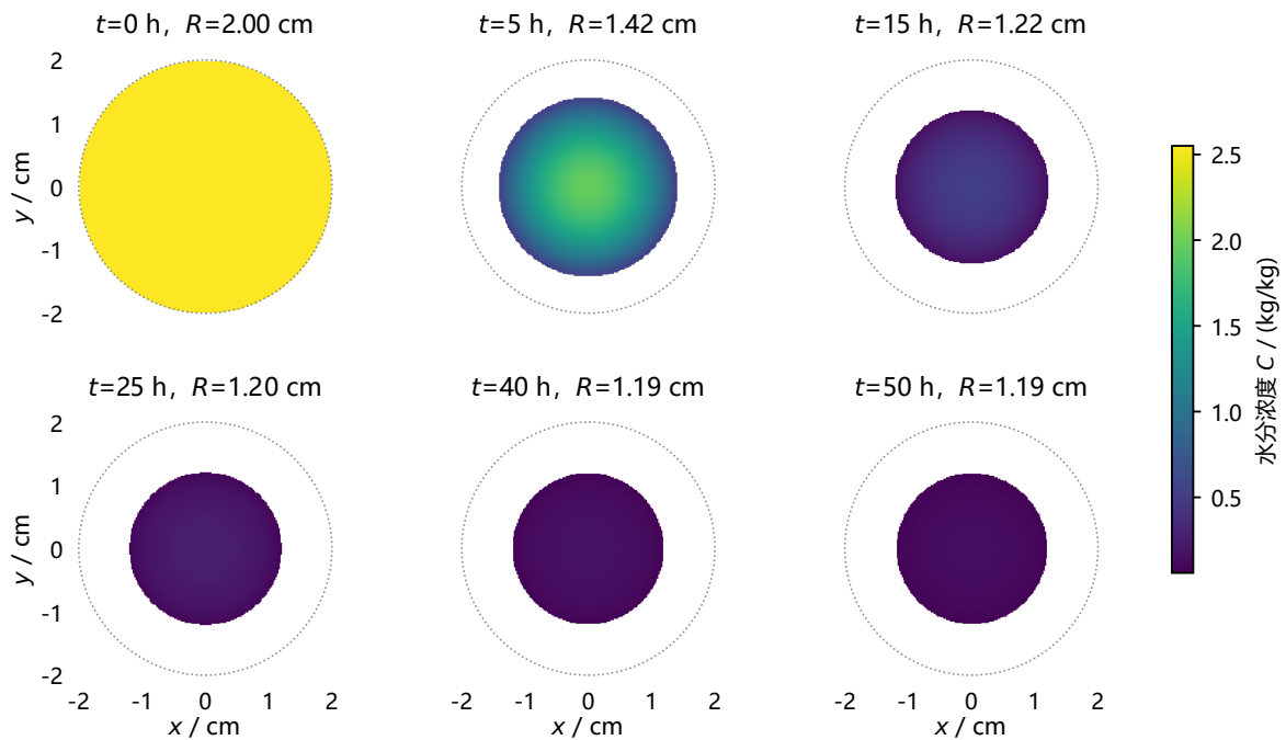
图 12 问题 4 的截面演化（回答“达标过程如何推进”）：6 个代表时刻的径向剖面热图，干燥自表面向中心推进、外半径同步收缩至平台 1.198 cm 附近（内生预测 1.19 cm）；中心为最慢点， t_f = 50.5369 h 时中心首次低于 0.15 kg/kg。
