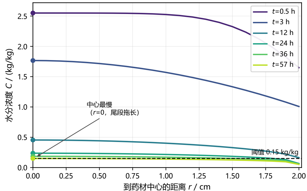
(b) 水分剖面 C(r, t) : 中心最慢、尾段拖长
