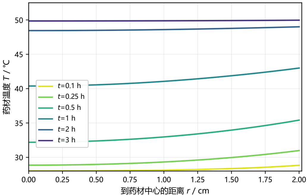
(a) 温度剖面 T(r, t) : 预热平衡 3 h 内即达准稳态
