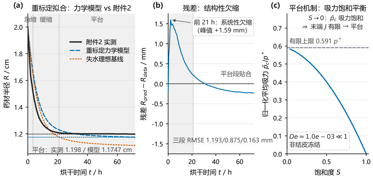
图 12 力学驱动内生收缩模型：修复后求解器 + 幂律保水重标定（ \beta = 0.106 ）对附件 2 的拟合结果为 RMSE 0.522 mm（残差三段：急缩 1.193 / 缓缩 0.875 / 平台 0.163 mm）、 t_f = 51.1667 h；末端 60–72 h 仅再降 0.04 mm（真平台），平台机制为吸力饱和平衡（ De \approx 10^{-3} \ll 1 ）。(c) 面板给出该平台机制：归一化平均吸力 \bar{p}_c/p^* 随饱和度 S 下降而单调上升，并在 S \rightarrow 0 时趋于有限上限 p^*/[(1 - \beta)(2 - \beta)] ——末端收缩进入平台即来自这一吸力饱和平衡；气相体积份额全程非负（ g_{\min} = 0.1446 ，无任何负孔隙）见表 3。
