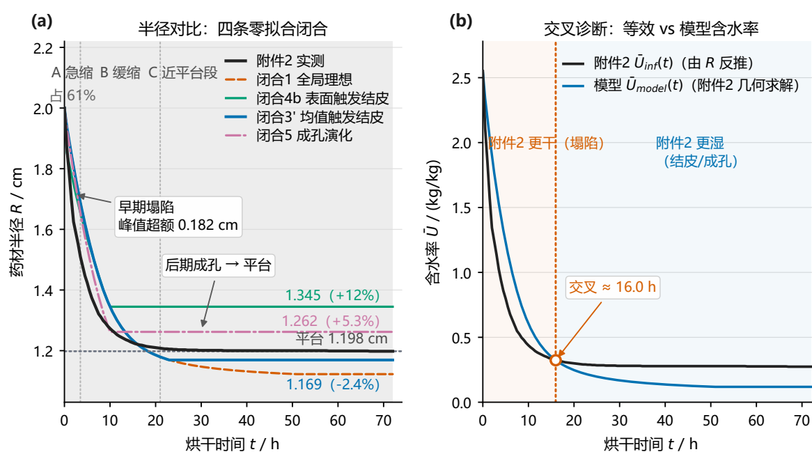
图8 附件2的收缩机制分析。附件2呈三段复合结构(A急缩61%/B缓缩/C近平台),与约16 h滞后交叉;零拟合的”理想收缩+玻璃化冻结”半经验闭合已能结构性给出减速与平台(均值触发那一条:平台1.169 cm、偏差-2.4%、冻结时刻偏差+12%),早期塌陷与后期成孔对应两组机制。数据源:问题4主解湿度场与附件2实测半径。
