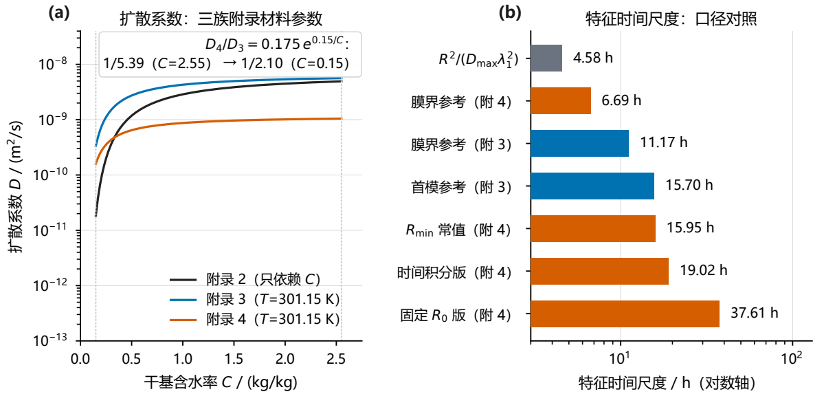
图 2 扩散系数非线性与特征时间尺度：(a) 三套附录材料参数的 D - C 半对数曲线——附录 2 只依赖 C 、不含 T ，附录 3/4 为 D(C, T) ；附录 4 全程低于附录 3，尾段 ( C \rightarrow 0.15 ) D 缩小 16.8 倍（该倍率按附录 3 材料参数公式算出、图上未单独标注）；(b) 各参考时标：常系数首模参考 15.7021 h、膜界 11.1720 h、问题 4 瞬时首模时间积分 19.016 h、固定 R_0 版 37.61 h、 R_{\min} 常值版 15.95 h——主值 57.18/50.54 h 均远大于各时标。
