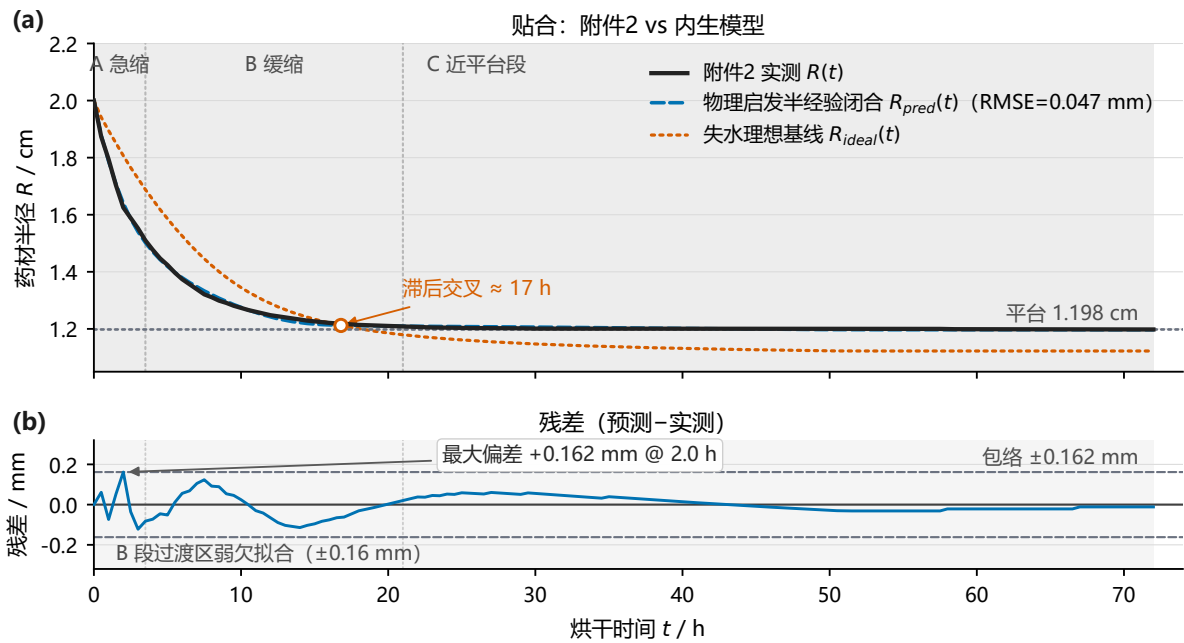
图 9 内生收缩模型对附件 2 的吻合与验证：式 (5.4) 由三项物理机制叠加而成，含 5 个标定参数与 2 个不参与拟合的量，它复现了附件 2 的全程形态：RMSE 0.047 \text{ mm} ，约为量化分辨率的 5 倍；滞后交叉 17.0 \text{ h} ，数据约 16 \text{ h} ；平台 1.1969 \text{ cm} ，数据 1.198 \text{ cm} ；三段形态全部复现。残差子图显示偏差始终在 \pm 0.16 \text{ mm} 以内，这是以实测几何单向驱动得到的拟合指标。
