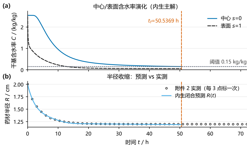
图 10 中心/表面含水率演化与半径收缩。(a) 中心与表面含水率曲线 + 0.15 kg/kg 阈值虚线 + t_f = 50.5369 h 达标竖线：表面先到干态、中心最后达标；(b) 内生半径 R(t) 在 50.5 h 进入近平台，60–72 h 仅再降 0.031 mm（模型已积分至 72 h，曲线止于 t_f = 50.54 h）。
