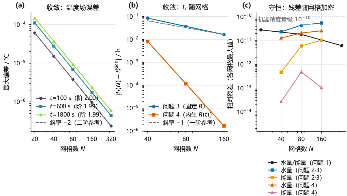
图 14 收敛与守恒检验。(a) 收敛·温度场误差：解析比较偏差随网格的二阶下降 (V1/V6); (b) 收敛· t_f 随网格的收敛序列; (c) 守恒·残差随网格加密：水量与显热离散平衡残差维持在 10^{-11} 量级附近 (V4)。
