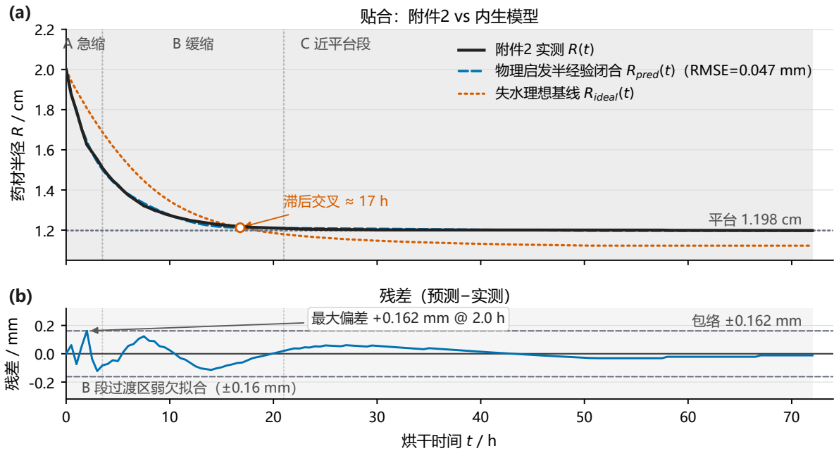
图 9 内生收缩模型对附件 2 的贴合与验证：三项物理动机机制的半经验闭合（式 (5.4)，5 个标定参数 + 2 个非拟合量）复现附件 2 的全程形态：RMSE 0.047 mm（量化分辨率的 5 倍）、滞后交叉（17.0 h vs 约 16 h）、平台（1.1969 vs 1.198 cm）、三段形态全对；残差子图显示偏差有界在 \pm 0.16 mm（单向拟合指标）。
