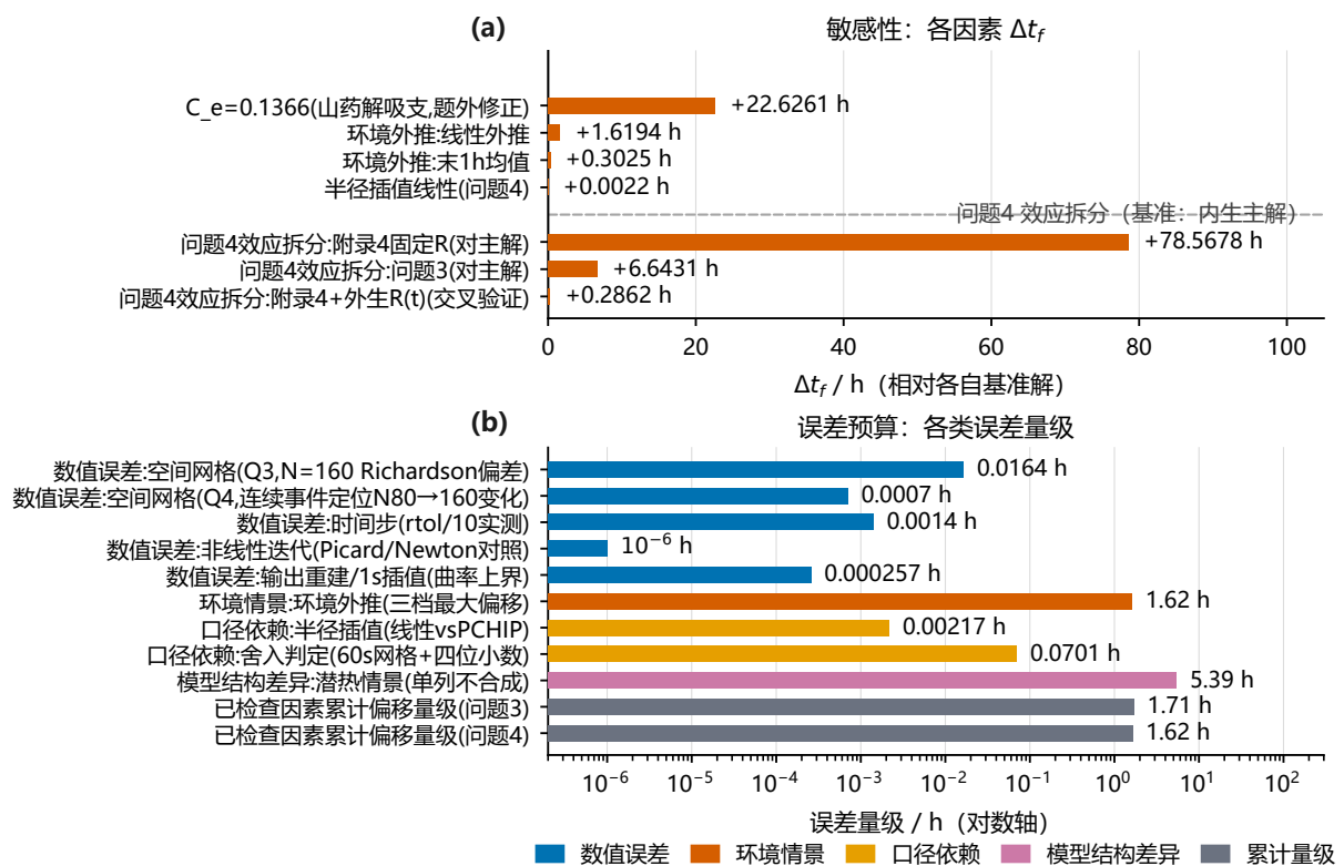
图 16 敏感性条形图: 各因素 \Delta t_f 横向条形, 边界汇取值 C_e = 0.1366 (题外修正) +22.63 h 自然主导, 环境外推 +1.62 h 次之, 半径插值仅 +0.002 h; 图中给出最大不确定性来源, 主结果一律用声明的闭合设定。
