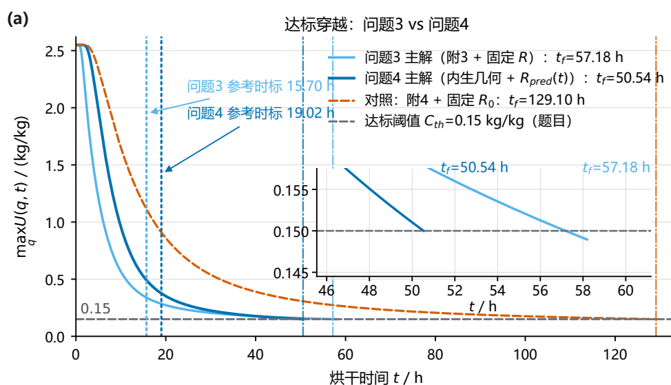
图 15 达标穿越： \max_q U(q, t) 全程曲线与 0.15 阈值线；问题 3 主解（ t_f = 57.1799 h）、问题 4 主解（ t_f = 50.5369 h，内生几何）与附录 4 固定半径对照（129.1047 h）三线对比，横轴标出参考时标（15.70 h / 19.02 h，常系数/瞬时首模近似，非严格误差界）。
