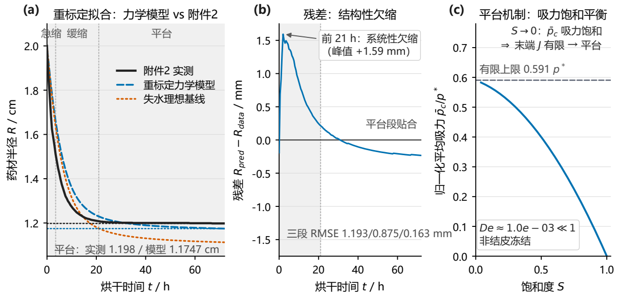
图 12 力学驱动内生收缩模型：修复后求解器 + 幂律保水重标定 ( \beta = 0.106 ) 对附件 2 的拟合结果为 RMSE 0.522 mm (残差三段：急缩 1.193 / 缓缩 0.875 / 平台 0.163 mm)、 t_f = 51.1667 h；末端 60–72 h 仅再降 0.04 mm (真平台)，平台机制为吸力饱和平衡 ( De \approx 10^{-3} \ll 1 )。(c) 面板给出该平台机制：归一化平均吸力 \bar{p}_c/p^* 随饱和度 S 下降而单调上升，并在 S \rightarrow 0 时趋于有限上限 p^*/[(1-\beta)(2-\beta)] ——末端收缩进入平台即来自这一吸力饱和平衡；气相体积份额全程非负 ( g_{\min} = 0.1446 ，无任何负孔隙) 见表 3。
