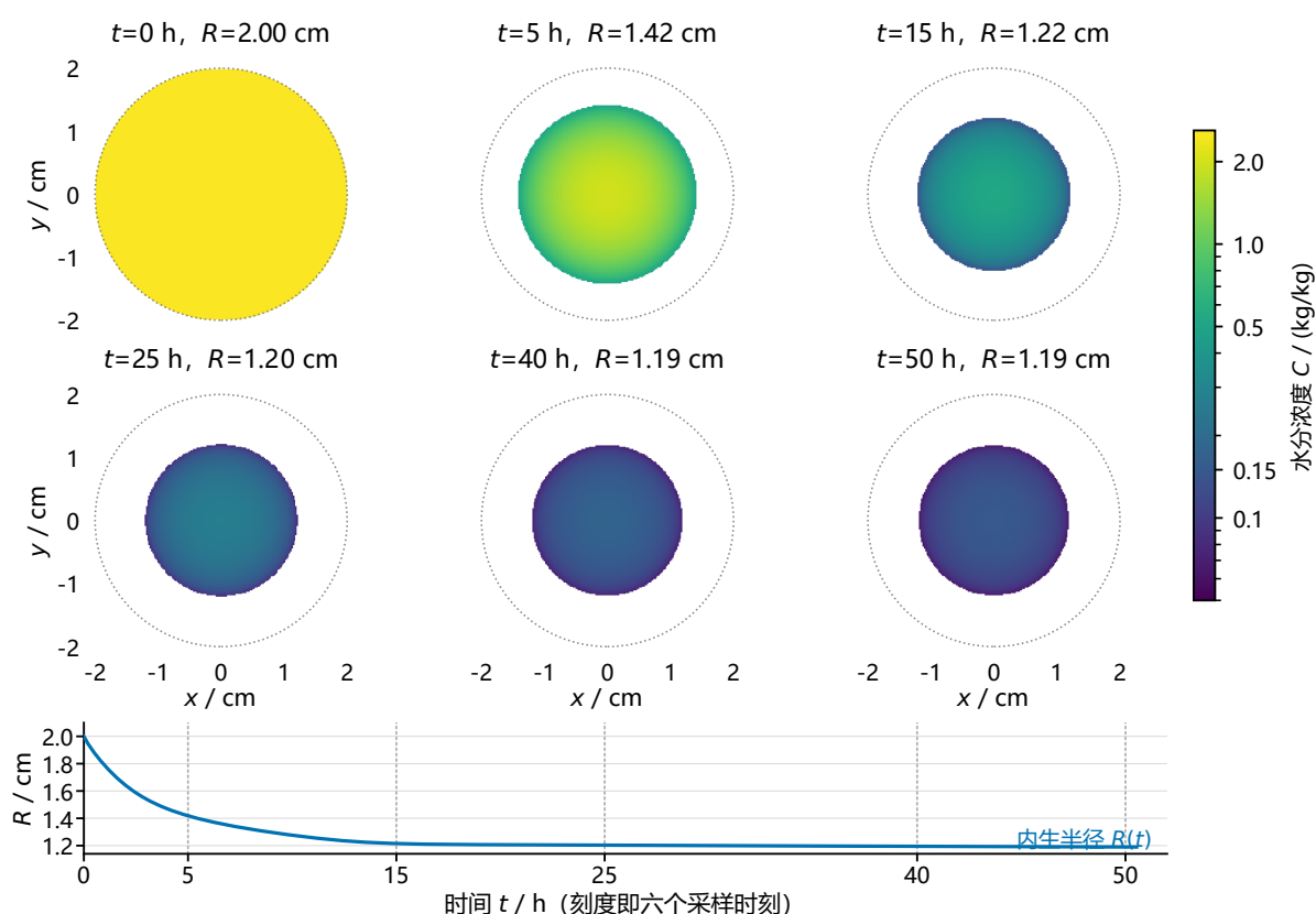
图 11 问题 4 的截面演化。6 个代表时刻的圆盘截面热图（色标为水分浓度，取对数色阶以便分辨低含水端的壳核差异，色标上 0.15 一刻即题目达标阈值）显示，干燥自表面向中心推进、外半径同步收缩并进入平台：附件 2 实测的平台半径为 1.198 cm，模型内生预测的末端半径为 1.19 cm（各面板标题给出该时刻的模型半径）；图底的时间轴带给出内生半径 R(t) 与六个采样时刻在曲线上的位置——六个盘的时间间隔是 5/10/10/15/10 h，而半径降幅集中在前两盘： R 在头 5 h 由 2.00 降到 1.42 cm（占总降幅 0.81 cm 的 72%），20 h 后即进入平台，故“等间隔取样、等宽排版”下视觉变化前快后慢；中心为最慢点， t_f = 50.5369 h 时中心首次低于 0.15 kg/kg。
