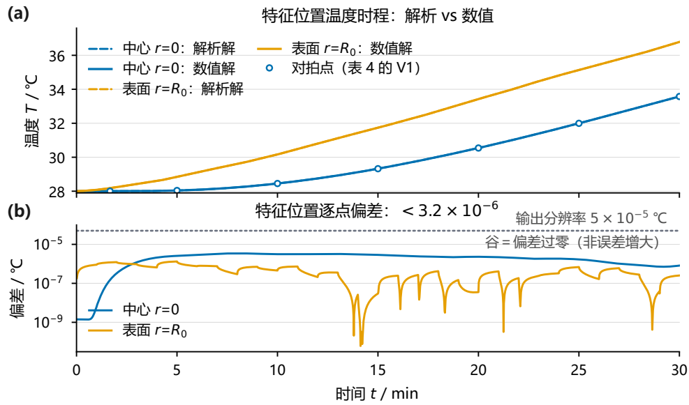
图 13 问题 1 解析比较 (V1): (a) 特征位置 (中心/表面) 温度的数值解与解析谱解时程; (b) 两个特征位置的逐点偏差时程, 量级 10^{-6} ^\circ\text{C} 、全程低于 3.2 \times 10^{-6} ^\circ\text{C} , 虚线为四位小数输出的分辨率上限; 径向网格加密的二阶收敛见表 5 与图 14(a); 全域单元中心在 N=320 的最大偏差为 5.9 \times 10^{-7} ^\circ\text{C} , 即正文引用的 V1 验证量。
