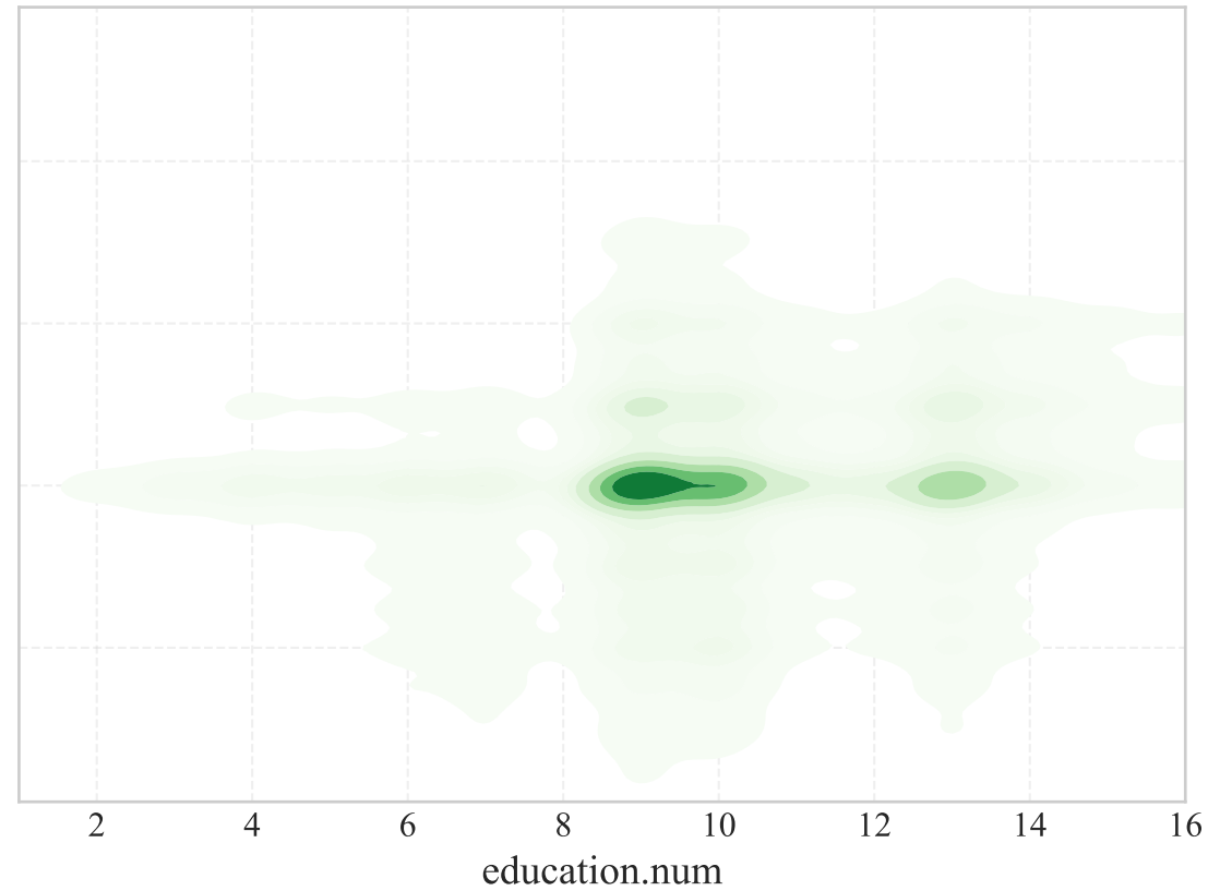
TAME (Ours)
