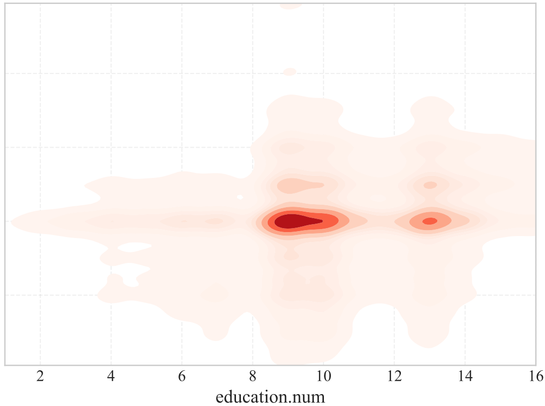
TabDDPM (Baseline)
