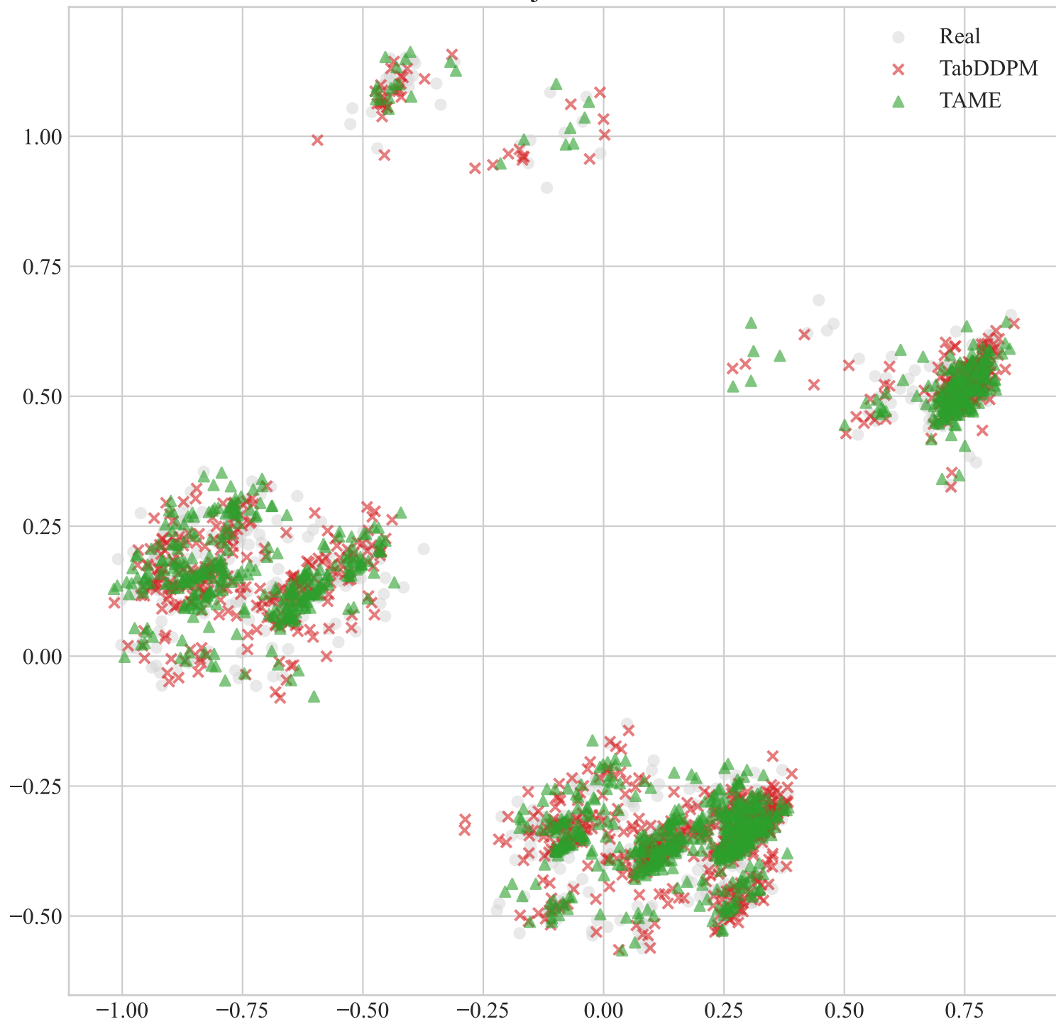
PCA Projection - adult
