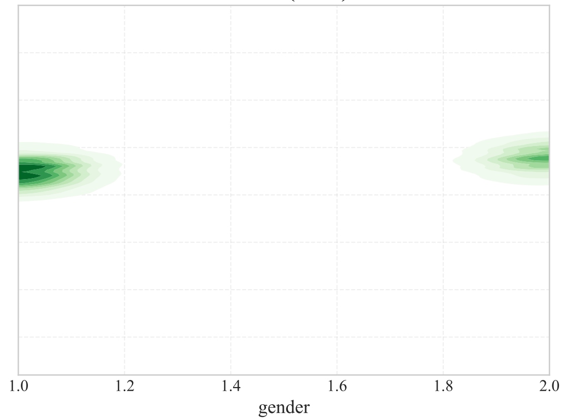
TAME (Ours)
