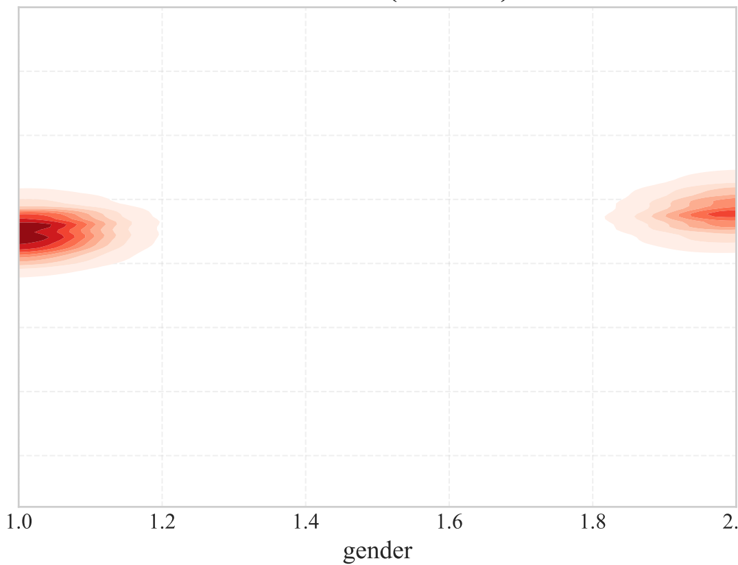
TabDDPM (Baseline)
