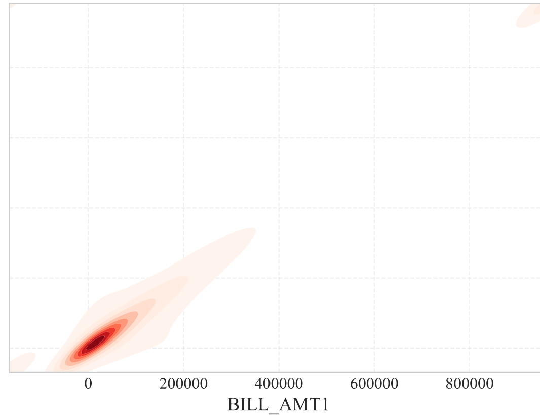
TabDDPM (Baseline)
