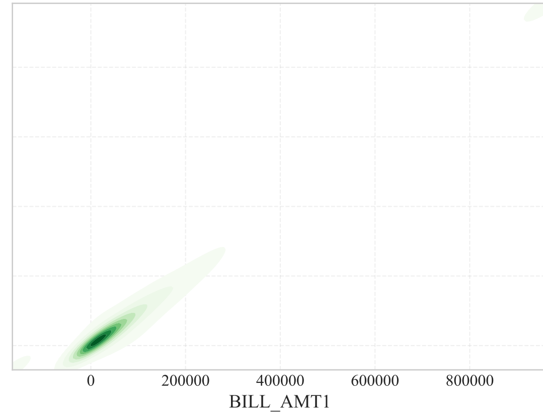
TAME (Ours)
