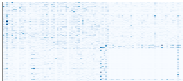
TabSyn +Tame
