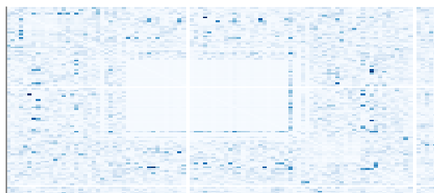
TabDDPM +Tame
