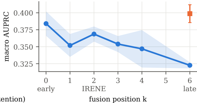
(b) Same sweep, macro AUPRC
