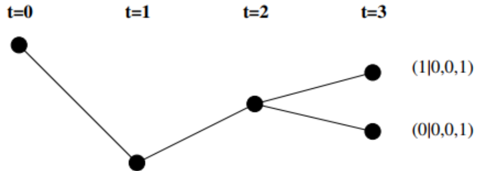
图 2.2: 两状态马尔科夫链的阿罗-德布鲁商品空间
