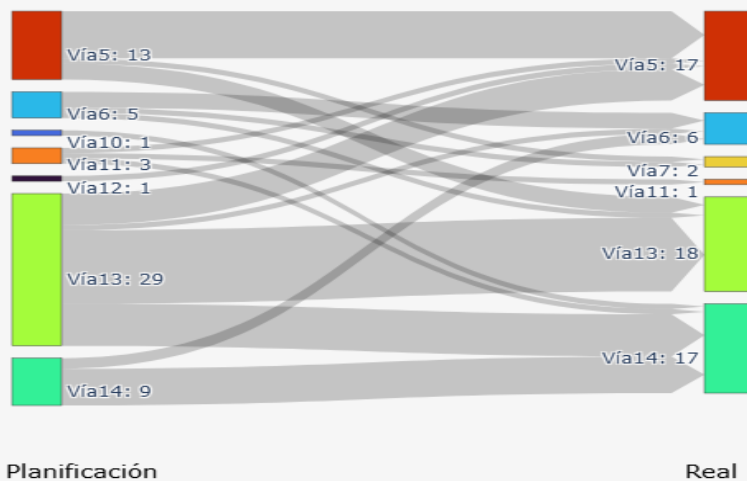
Planificación Vías ALACANT-TERMINAL (SD Este) 2025-09-21
