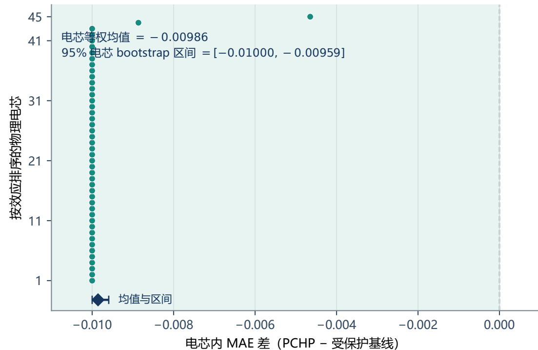
A 冻结外部确认：45/45 个电芯改善
