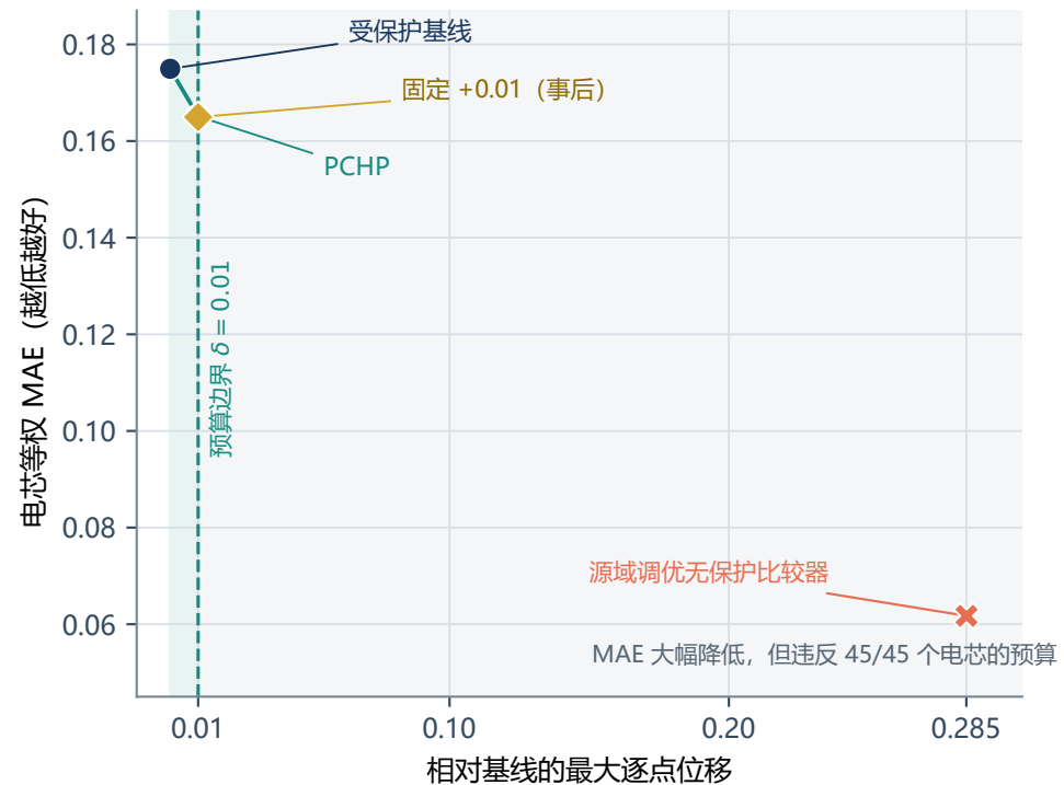
B 安全—精度边界
