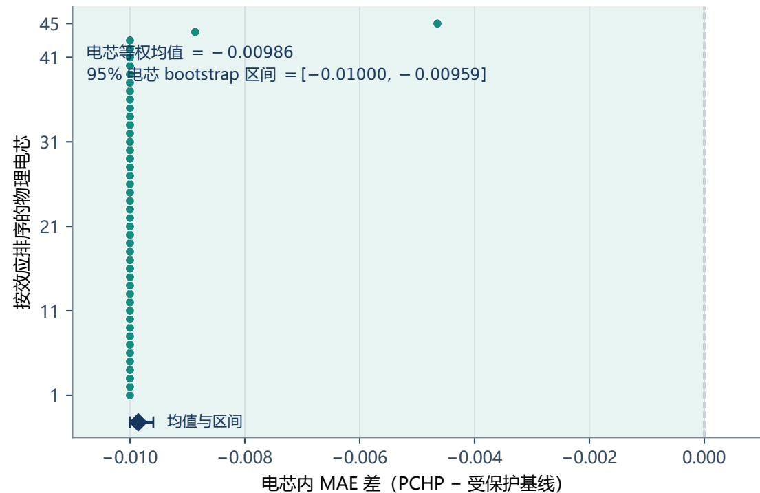
A 结果盲、协议锁定外部验证：45/45 个电芯改善
