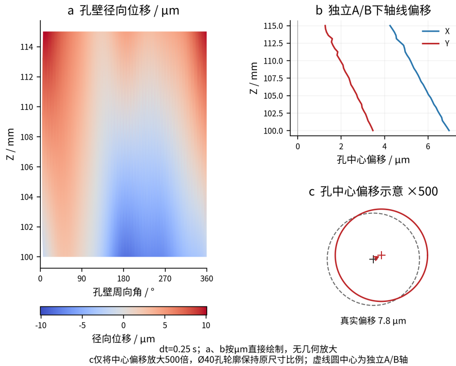
图7 完全卸夹孔区；h1.125、dt0.25；热残余直径15.6 \mu\text{m} ；左与右上按 \mu\text{m} 直接绘制，无几何放大；右下孔中心偏移示意 \times 500 ，孔轮廓保持原尺寸比例
