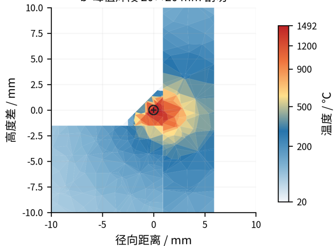
b 峰值焊段 20\times 20\text{ mm} 剖切
