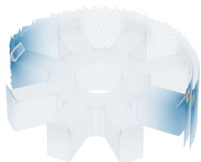
a 座体、壳体与焊段（壳体剖开）
