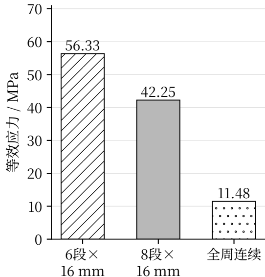
(a) 静载计算
