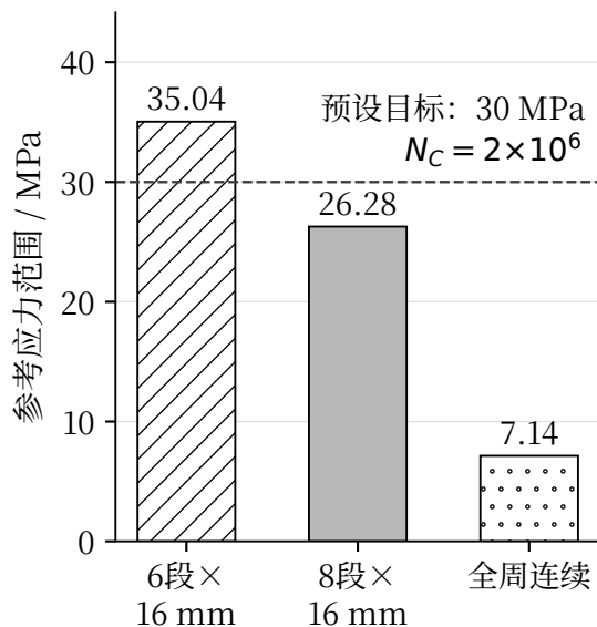
(b) 疲劳计算
