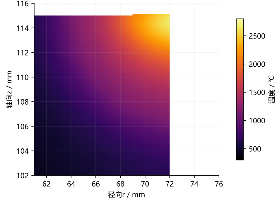
d t=9.641 s收弧截面实际温度
