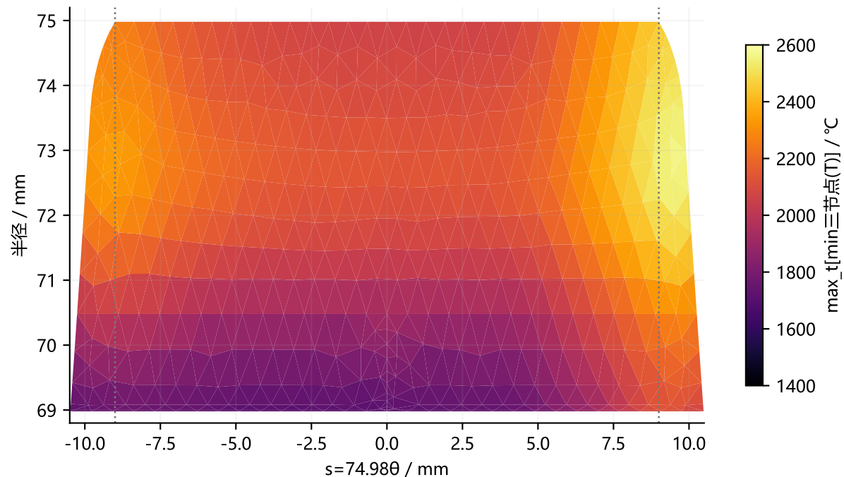
d t=9.641 s收弧截面实际温度
