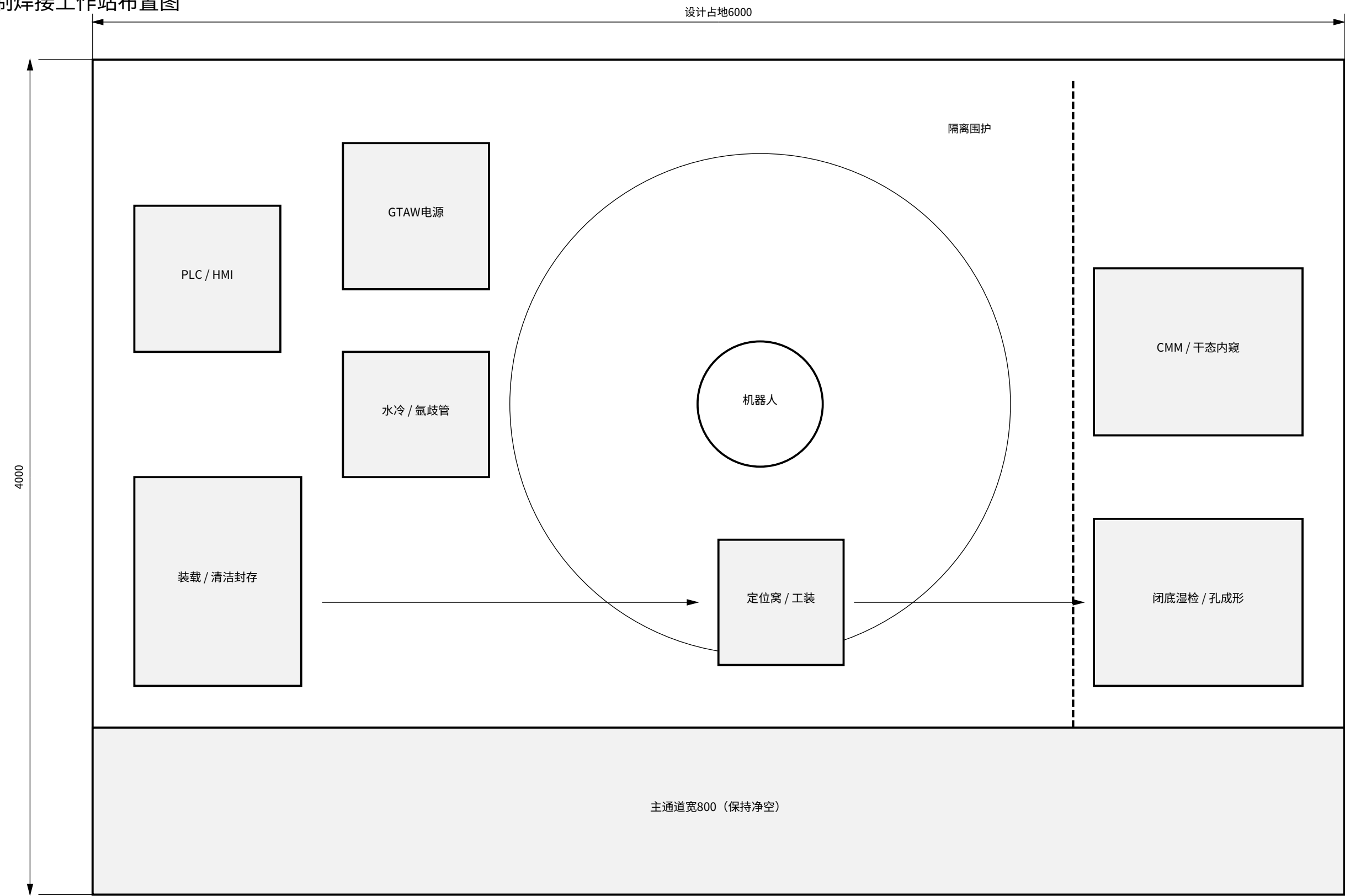
首批试制焊接工作站布置图
