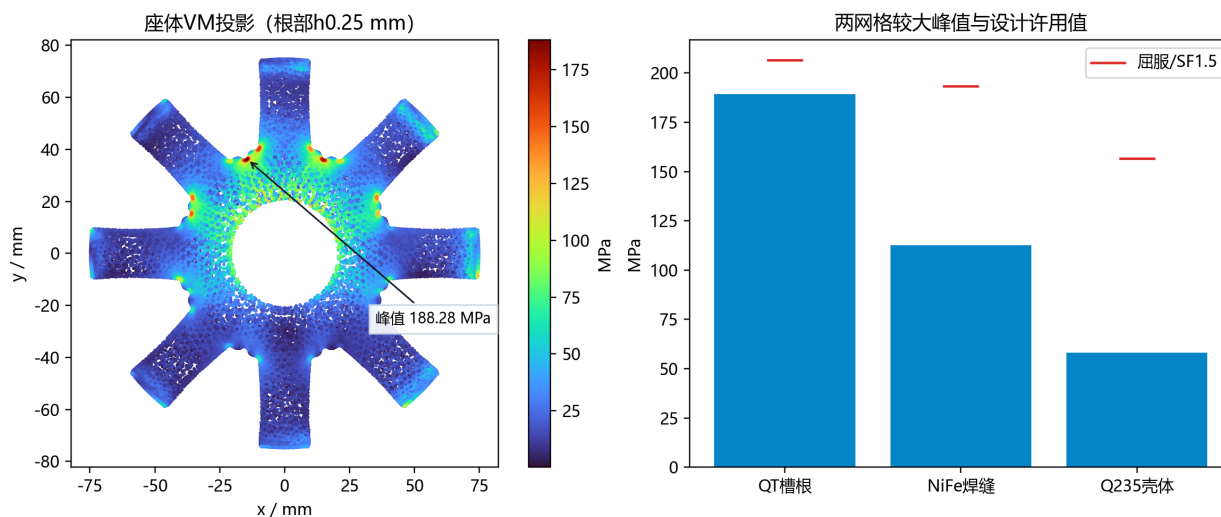
整件设定载荷应力场与许用值
