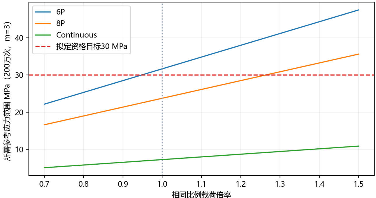
相同假定载荷谱下的疲劳敏感性
