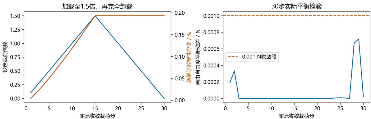
实际加载卸载塑性演化与平衡残差
