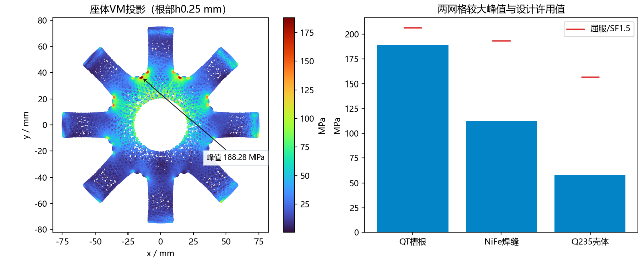
整件设定载荷应力场与许用值
