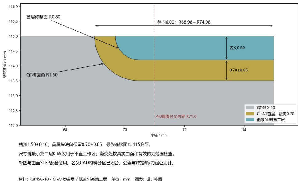
HJ-DRW-017 独立预制与首层曲面修整名义断面
