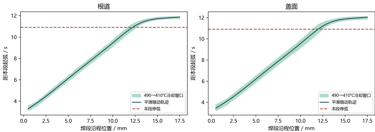
真实热场的轻击温窗与随动轨迹
