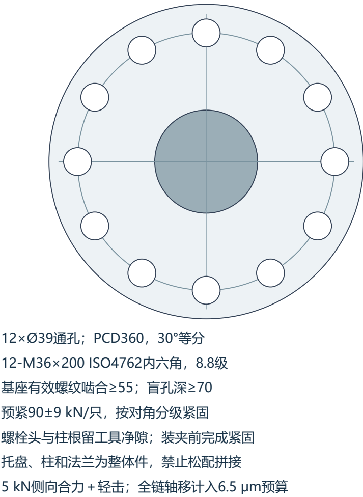
法兰俯视 (NTS)
