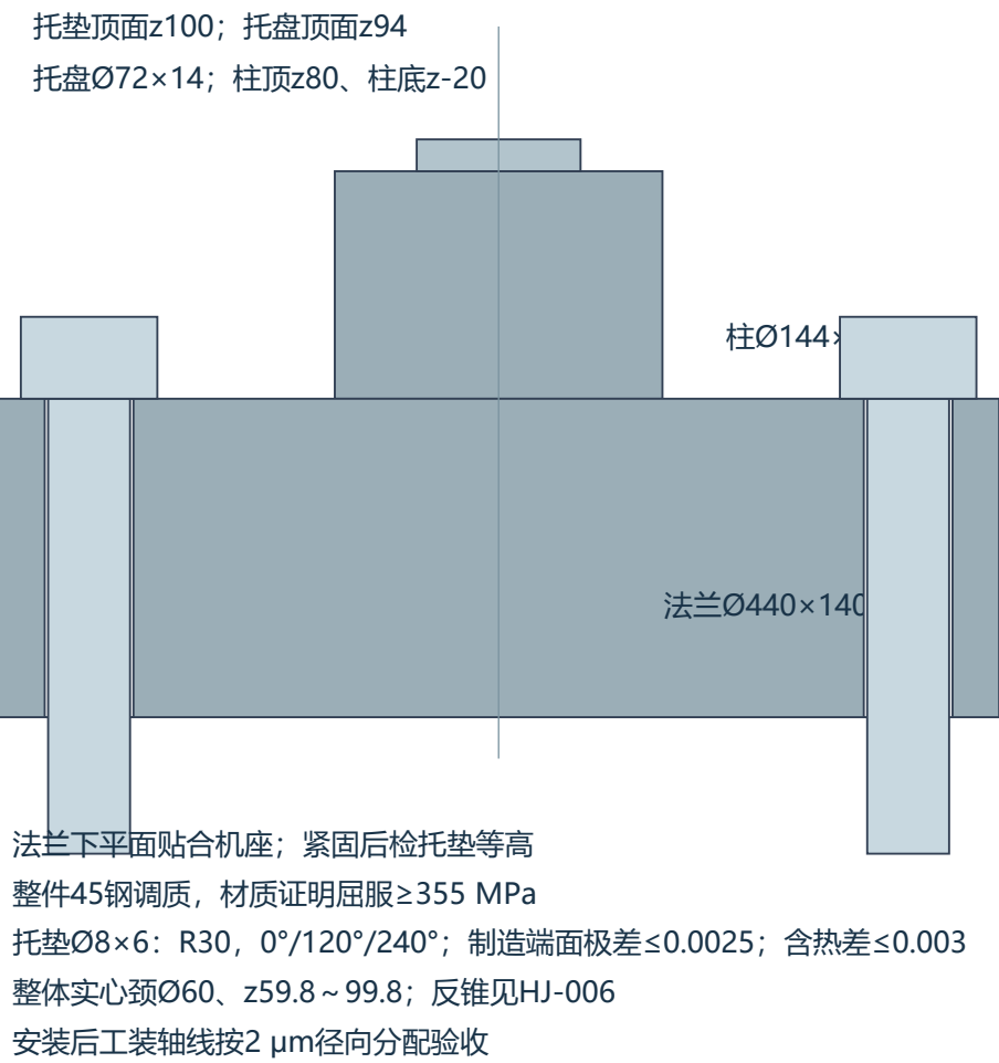
轴向剖面 (NTS)
