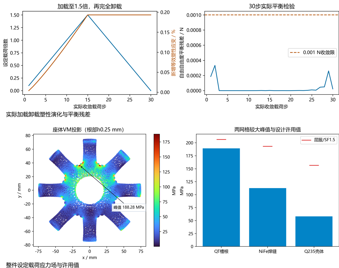
整件设定载荷应力场与许用值
