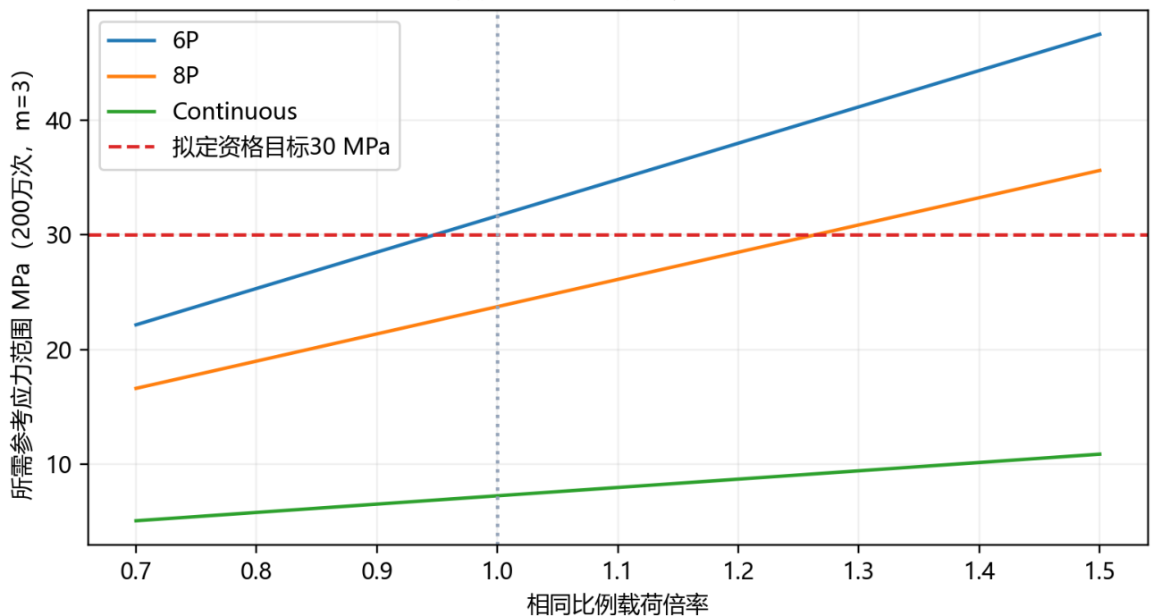
假定同谱下的疲劳资格要求
