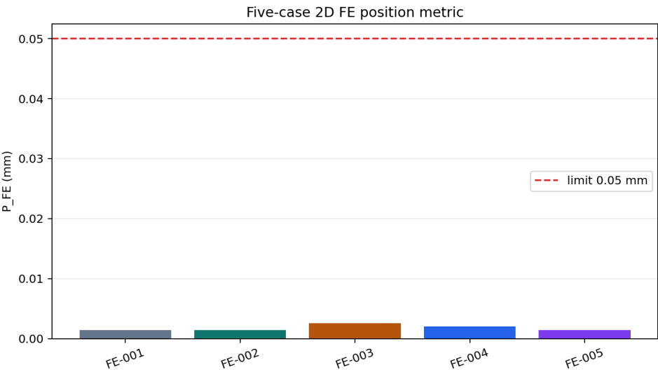
图 3 FE-001..005 的二维代理几何响应指标。来源：simulation/fe/results/fe-summary.csv。
