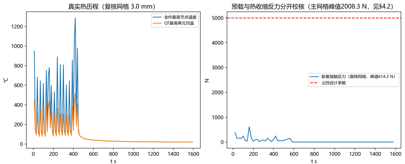
热历程与胀套接触反力
