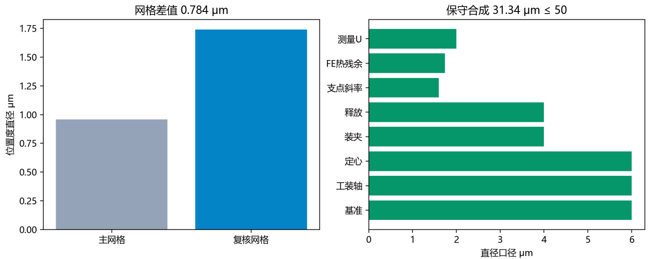
两网格位置度预算与差值
