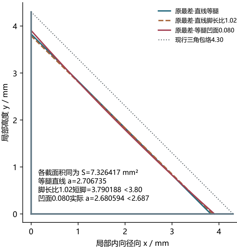
C 固定面积的合法截面：面积充足仍可短脚或喉部不足
