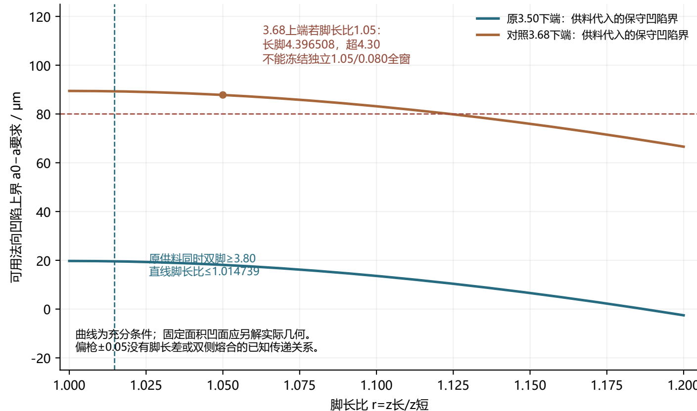
D 原包络与唯一供丝对照：保持4.30外包络
