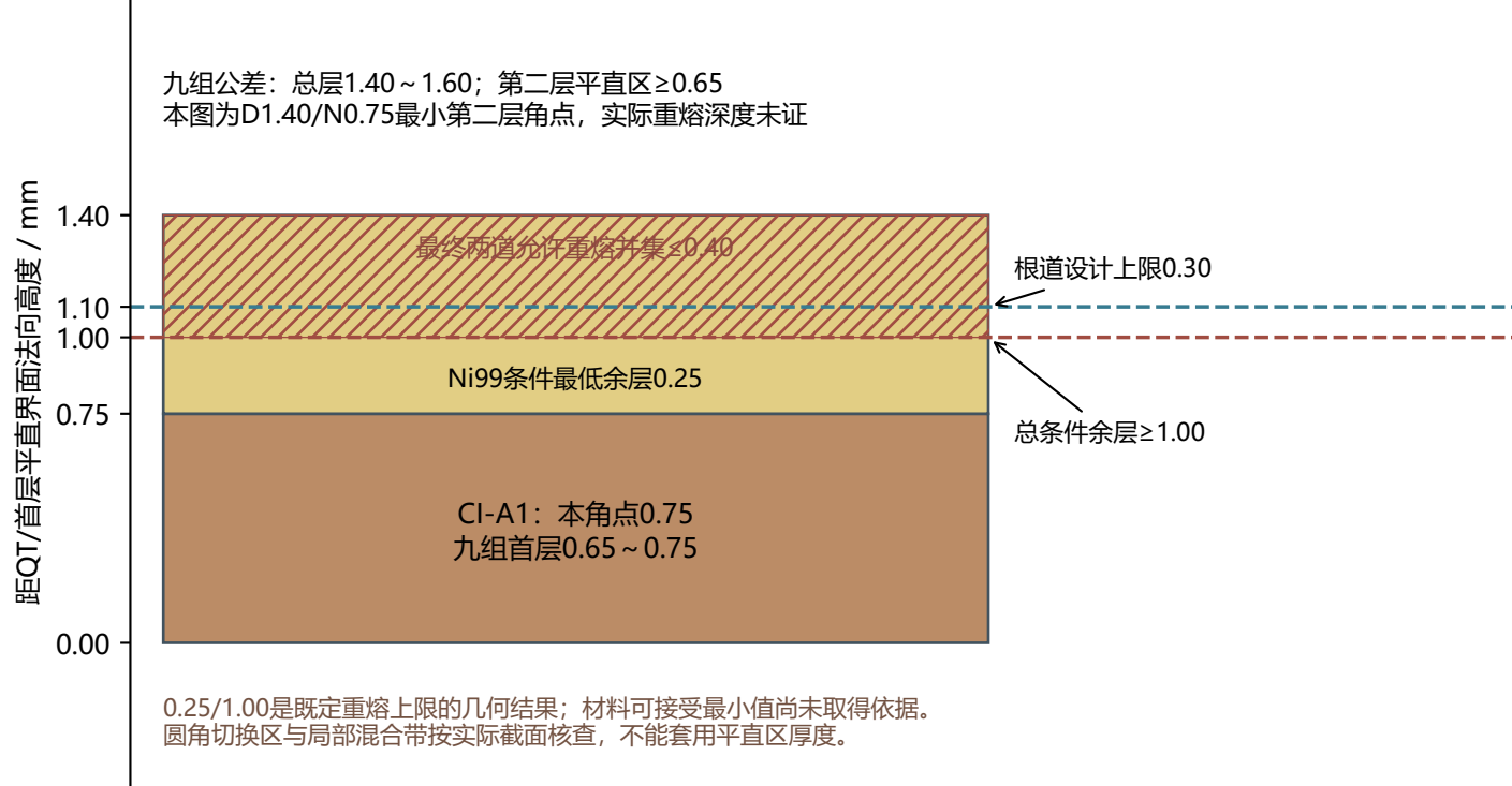
B 最低留层与重熔限值：条件几何关系
