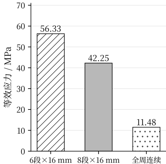
(a) 静载计算
