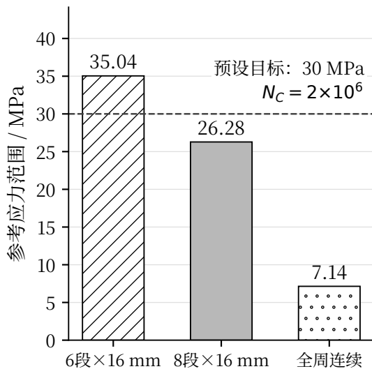
(b) 疲劳计算
