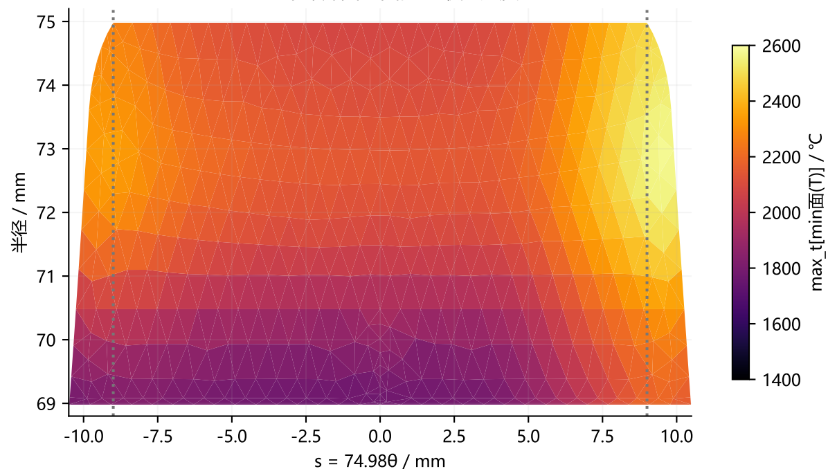
d 收弧 t=11.569 s端部截面瞬时温度
