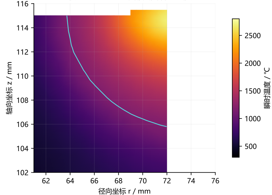
d 收弧 t=11.569 s端部截面瞬时温度
