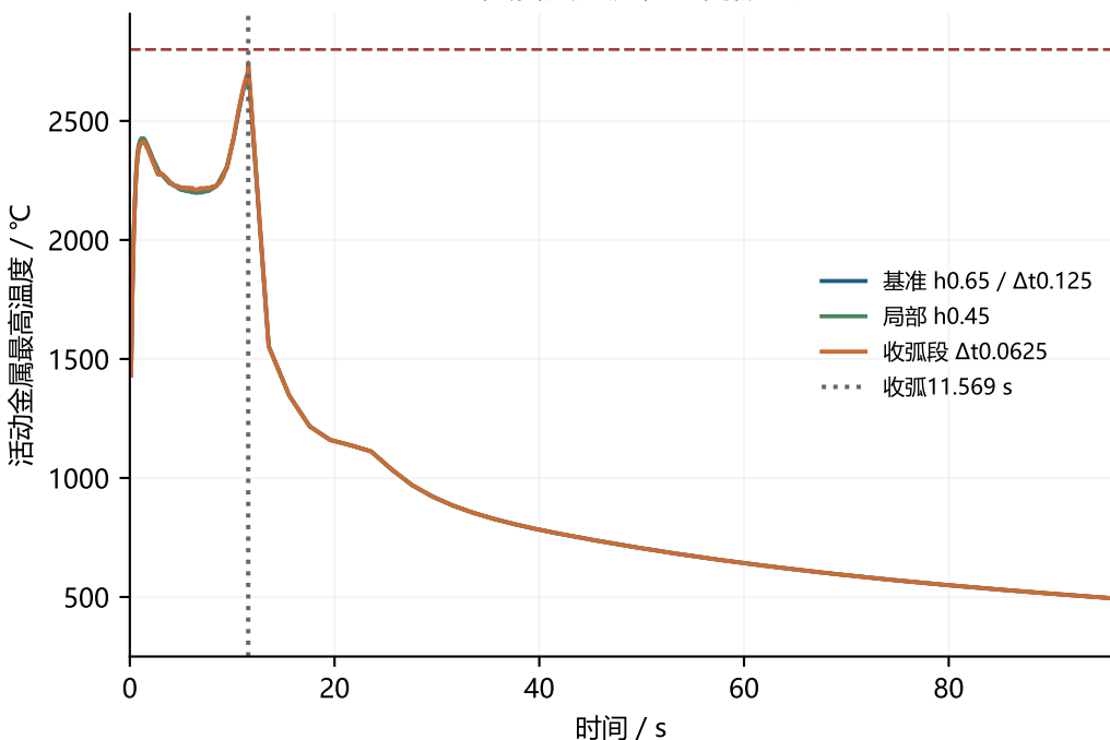
c 中央18 mm最弱面的热连接检查
