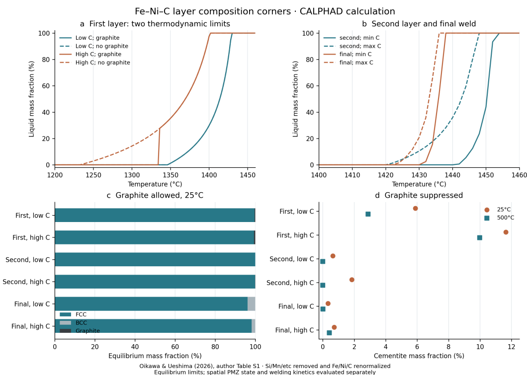
Fe-Ni-C各层成分角点与石墨条件计算
