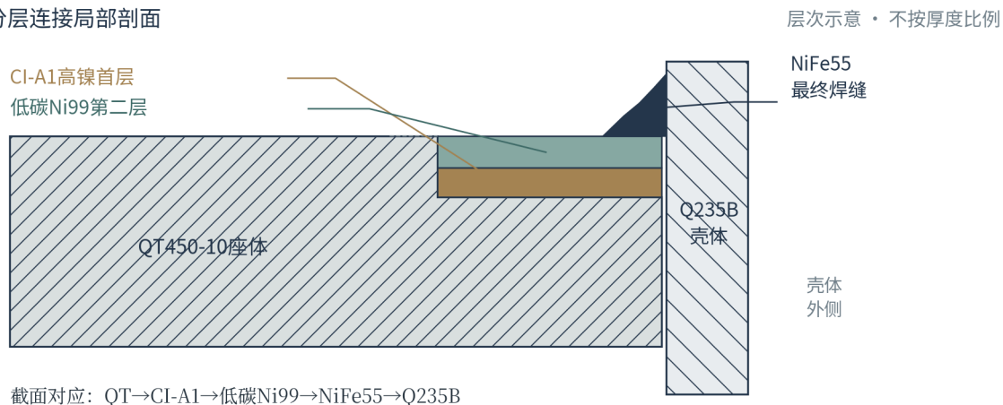
圆环分层连接局部剖面
