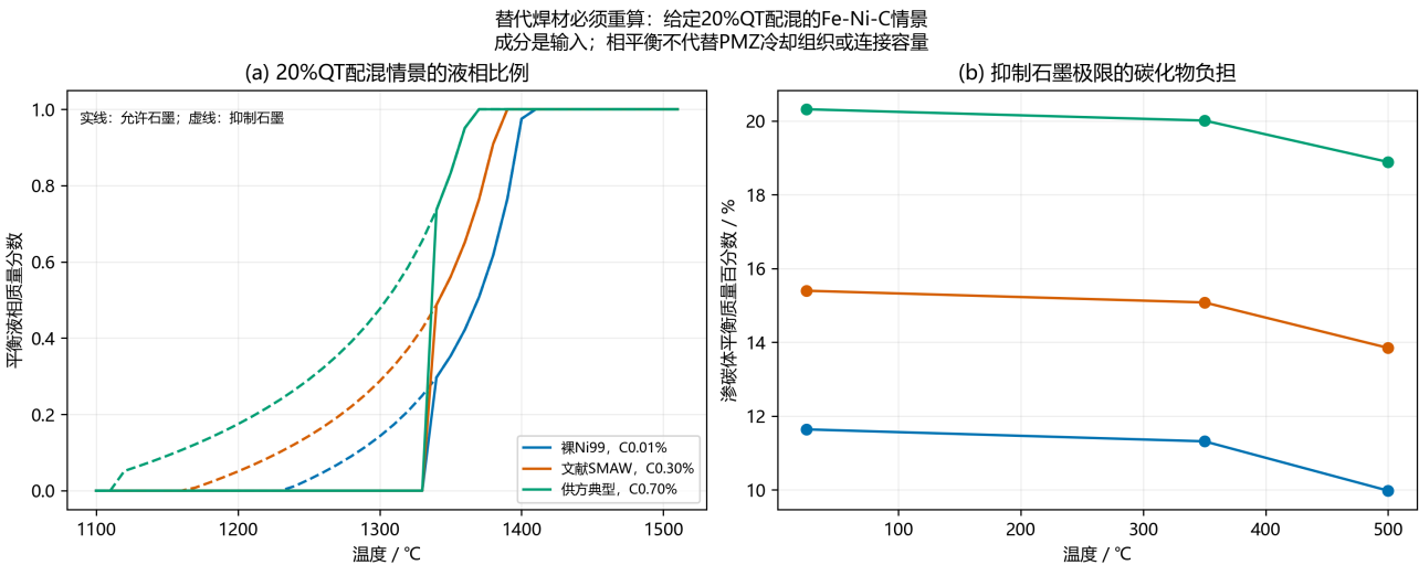
三类高镍焊材20%QT配混的实际相平衡比较
