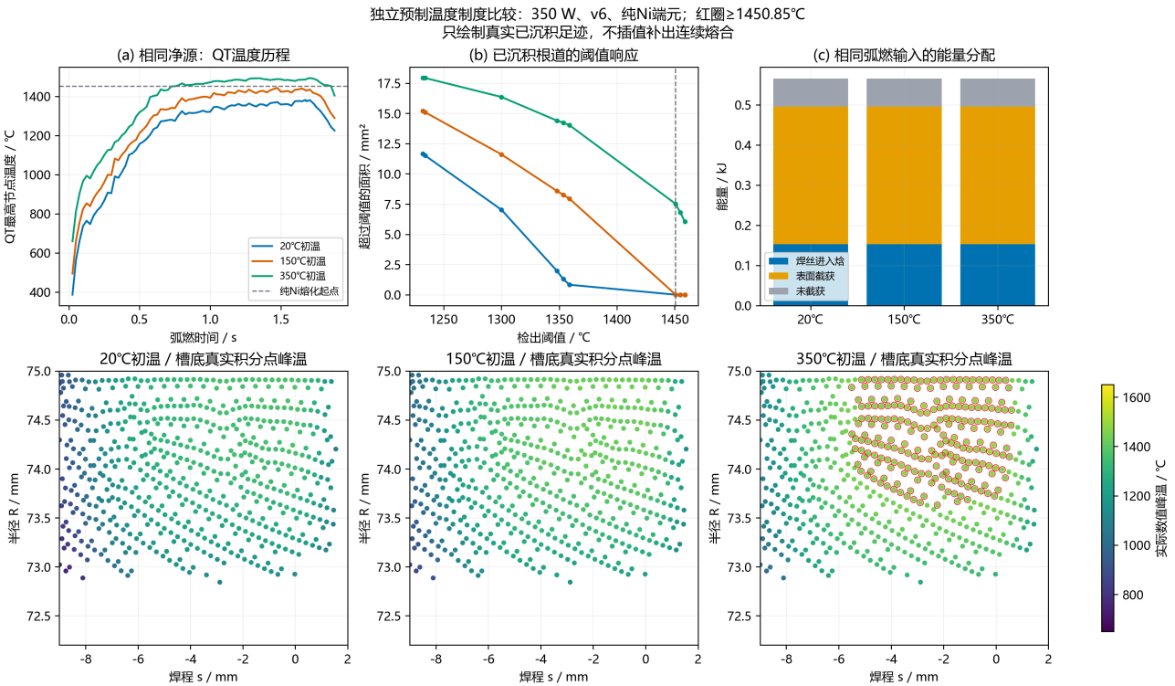
独立预制三档初温的实际热循环、阈值响应和根道峰温
