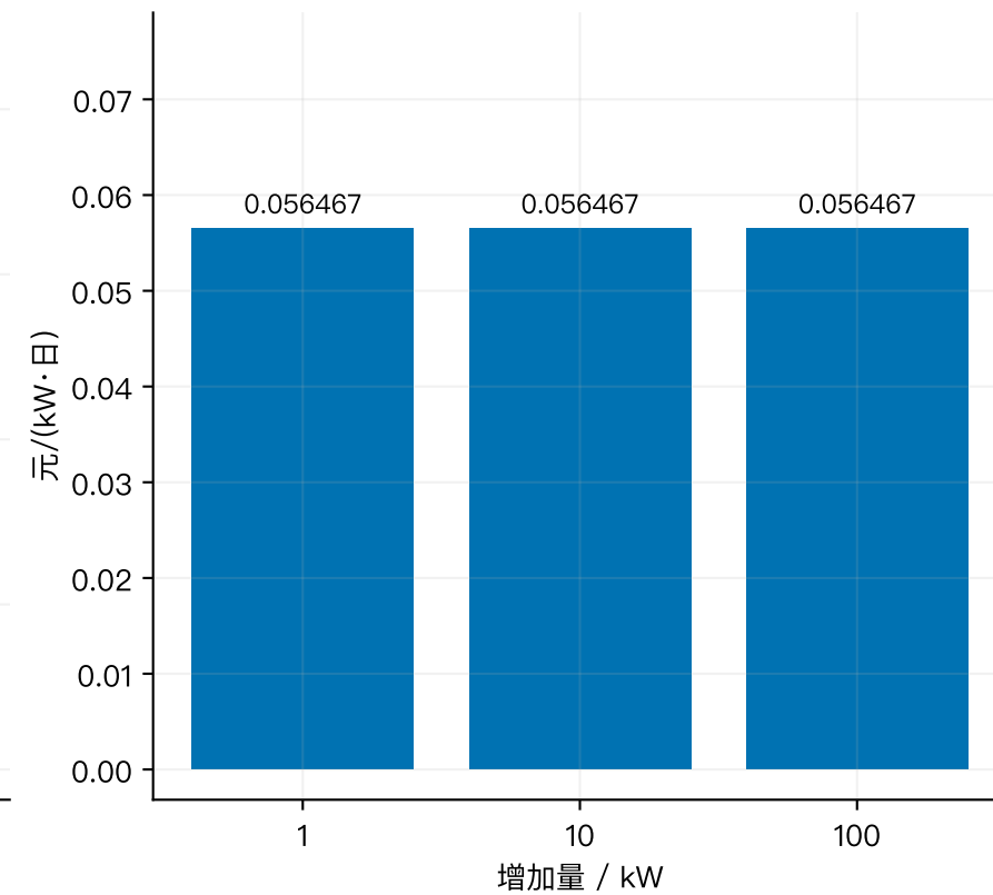
充电功率上限 基准活跃 19 个时段
