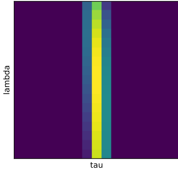
tau-lambda
