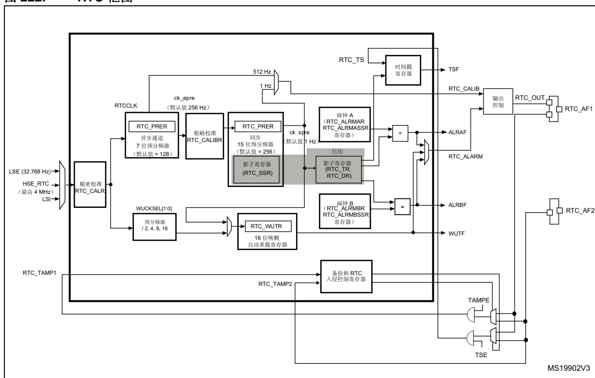
图 222. RTC 框图
