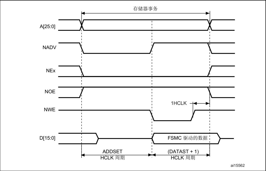
图 410. 模式 2 写入访问
