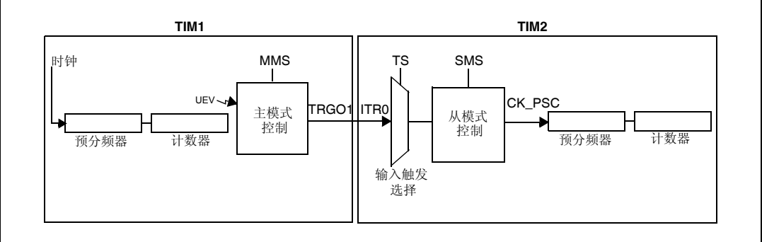
图 159. 主/从定时器示例
