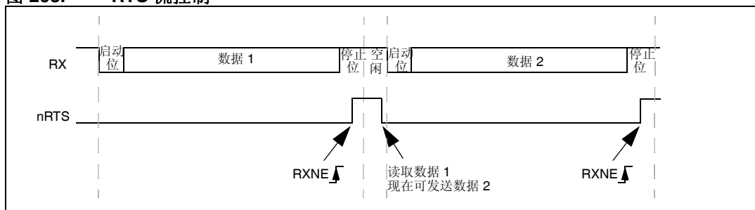
图 268. RTS 流控制
