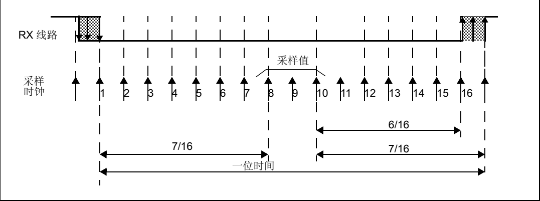
图 251. 16 倍过采样时的数据采样
