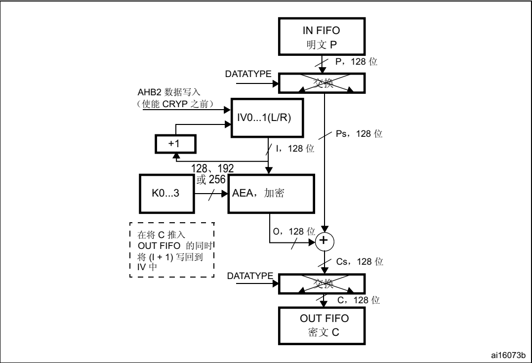
图 211. AES-CTR 模式加密
