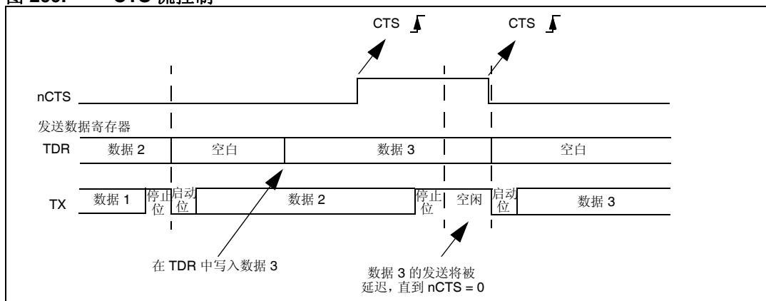
图 269. CTS 流控制
