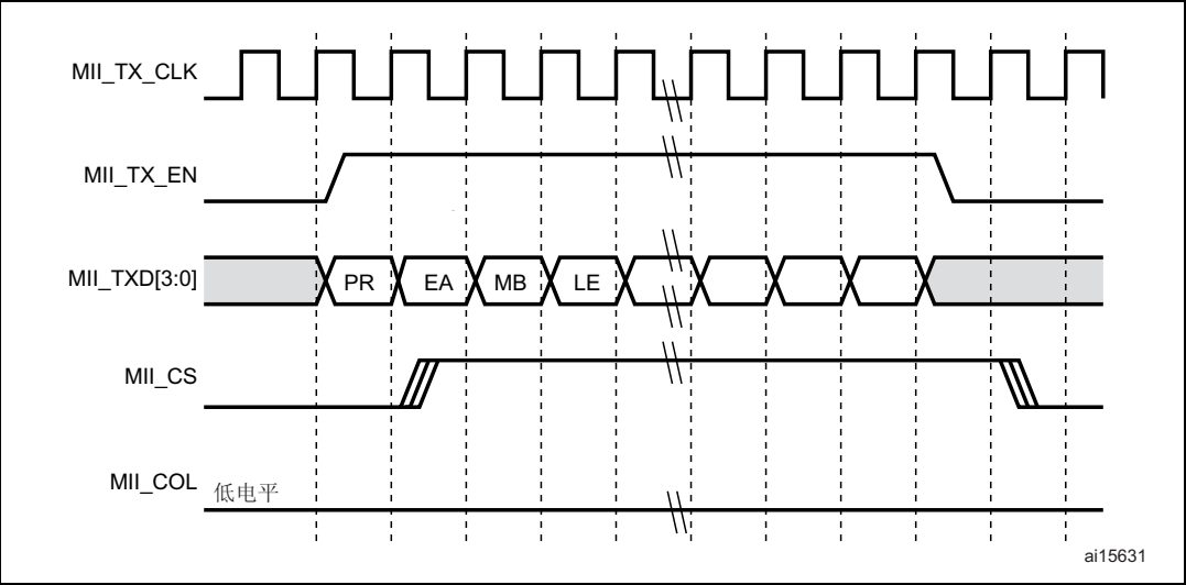
图 334. 无冲突发送
