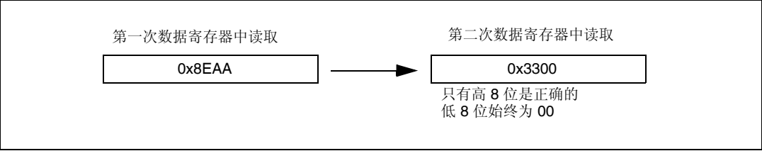
图 292. 接收 0x8EAA33
