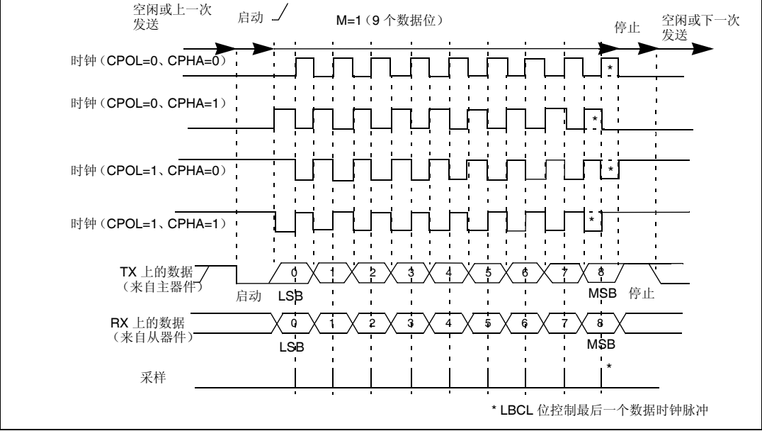
图 259. USART 数据时钟时序图 (M=1)
