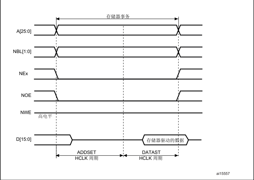
图 405. 模式 1 读取访问
