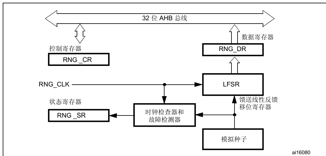
图 217. 框图
