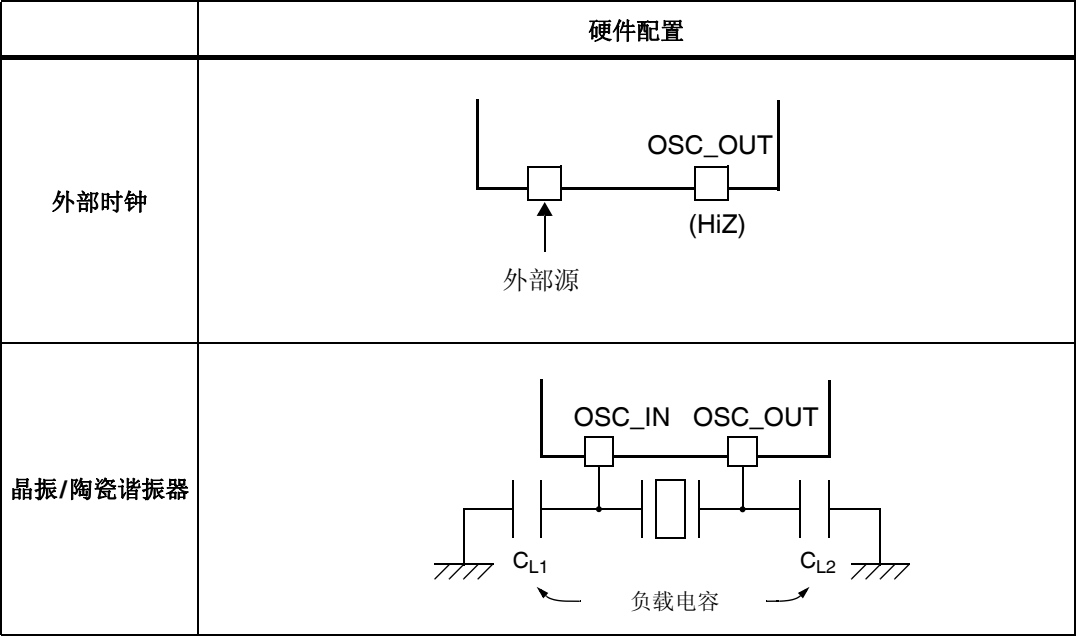
图 14. HSE/LSE 时钟源
