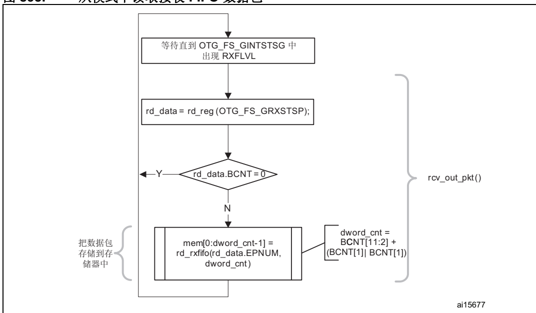
图 395. 从模式下读取接收 FIFO 数据包
