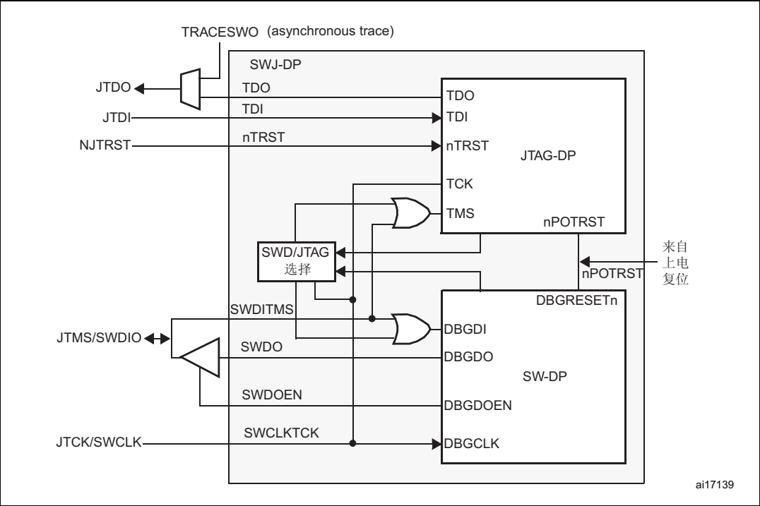
图 426 显示了异步 TRACE 输出 (TRACESWO) 与 TDO 复用。这意味着异步跟踪只能在 SW-DP 上实现，不能在 JTAG-DP 上实现。
