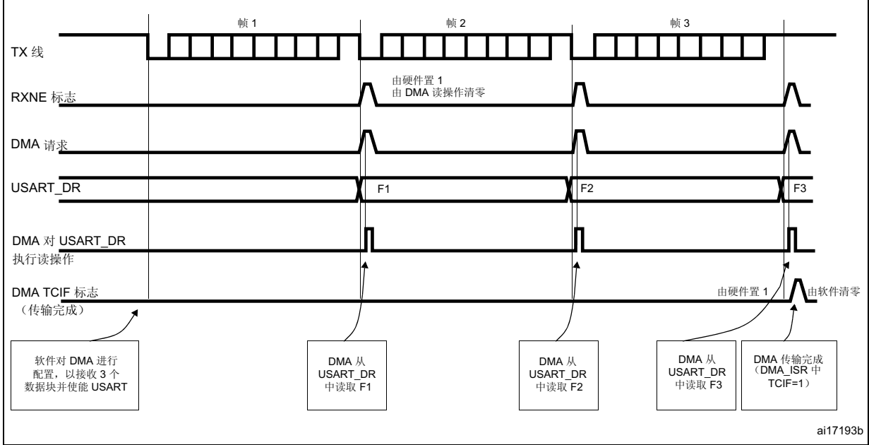
图 266. 使用 DMA 进行接收
