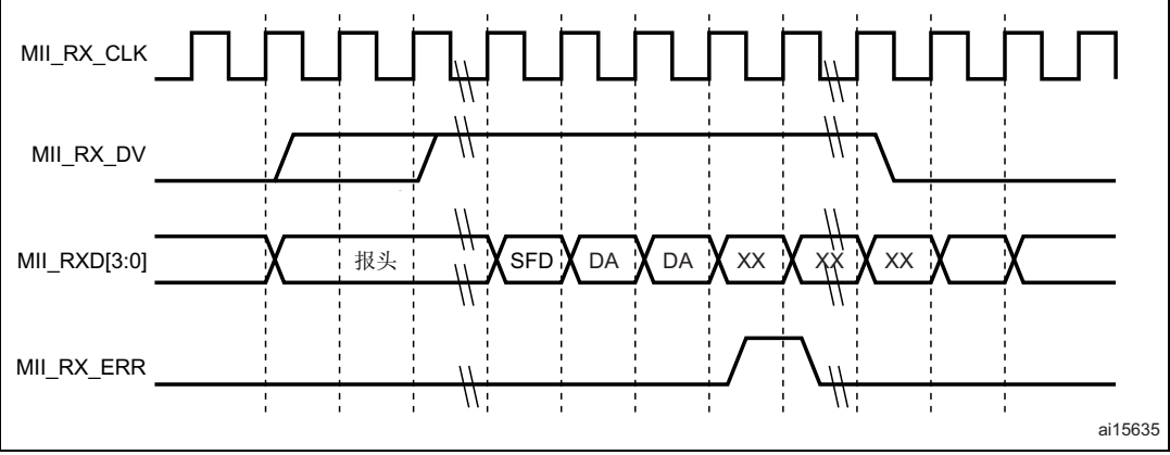
图 339. 有错误接收
