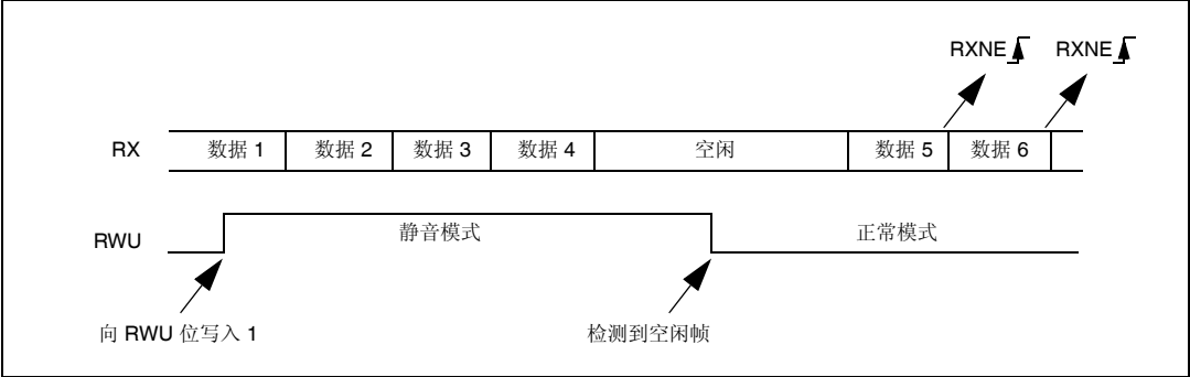
图 253. 使用空闲线路检测时的静音模式
