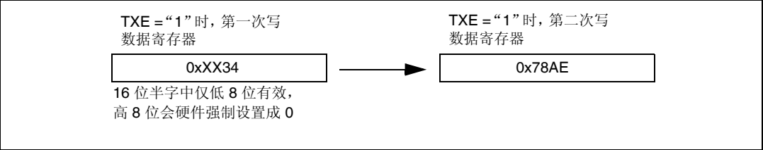
图 300. 发送 0x3478AE 所需的操作
