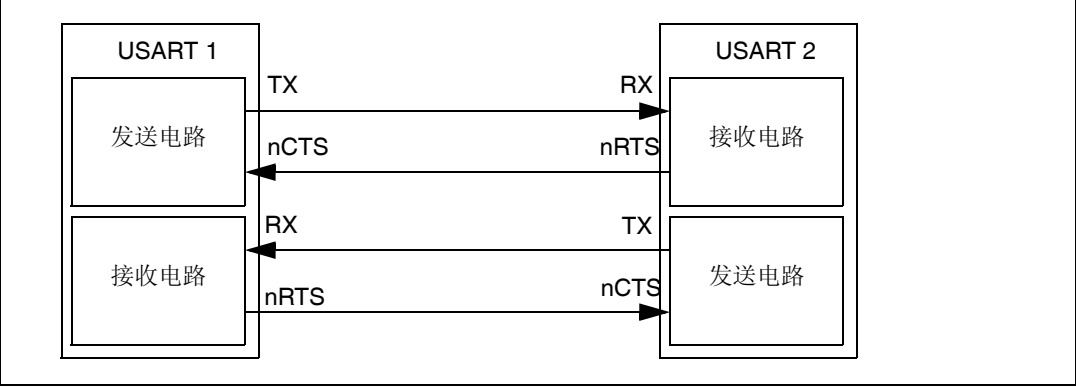
图 267. 2 个 USART 间的硬件流控制
