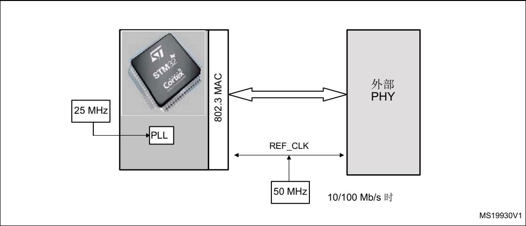
图 328. RMII 时钟源
