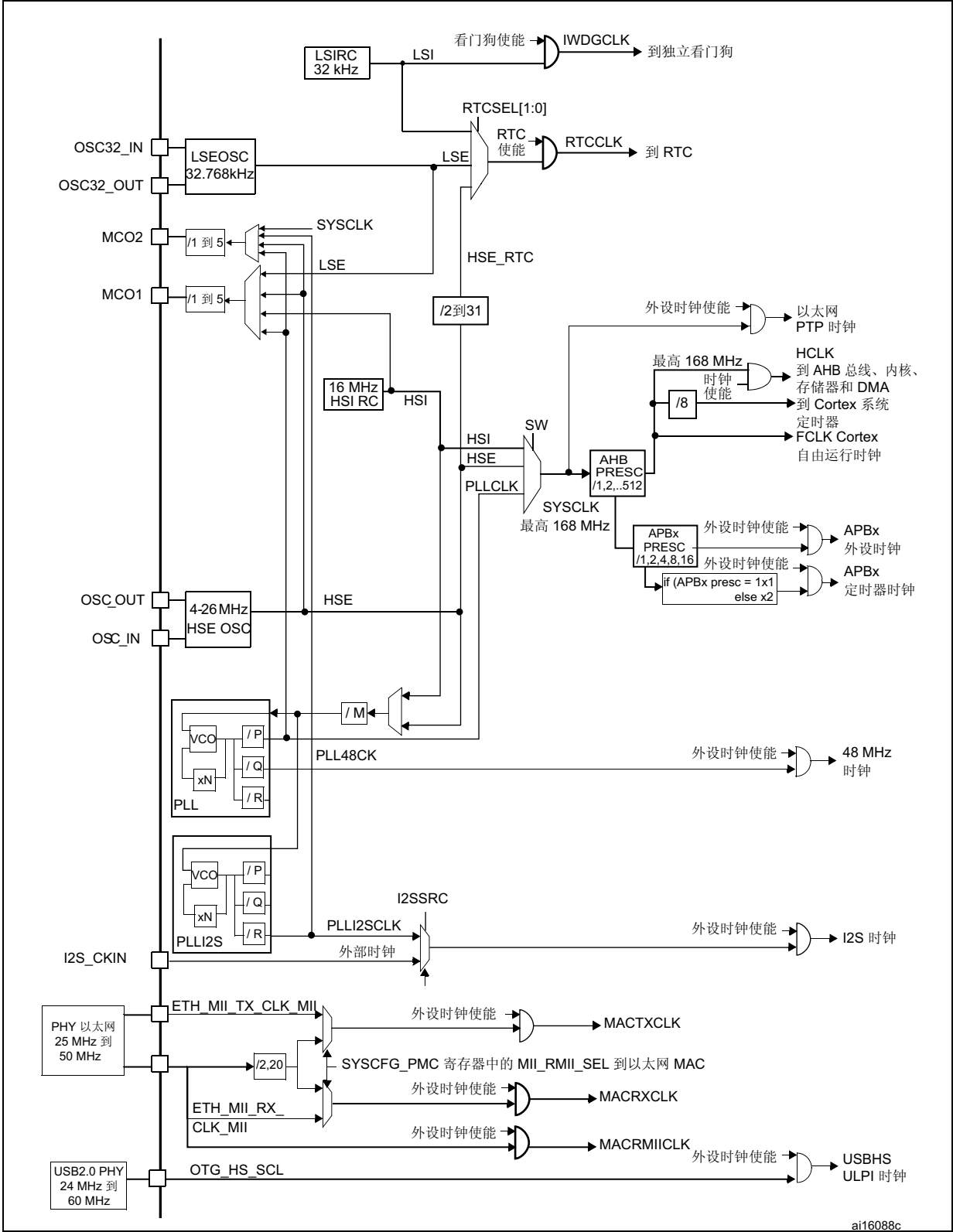
图 13. 时钟树
