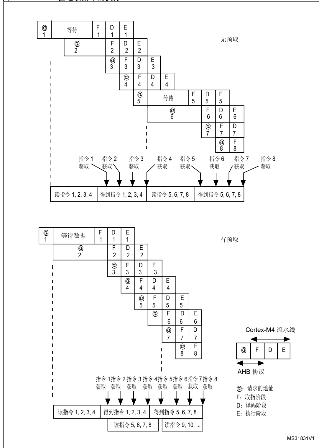
图 4. 32 位连续指令的执行
