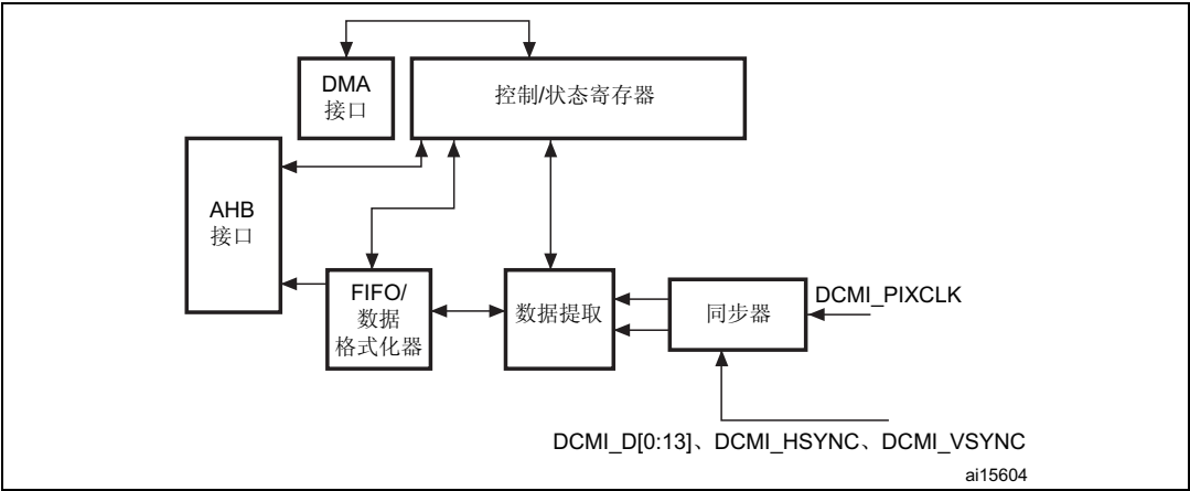
图 62. DCMI 框图
