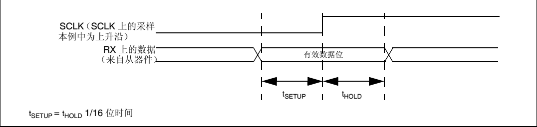
图 260. RX 数据建立/保持时间
