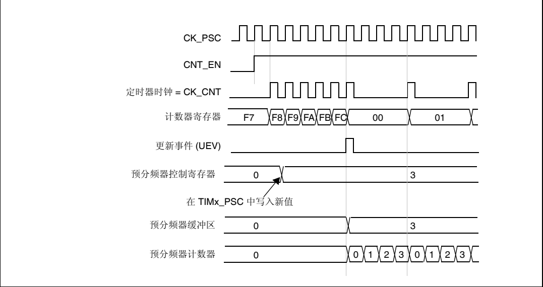
图 190. 预分频器分频由 1 变为 4 时的计数器时序图
