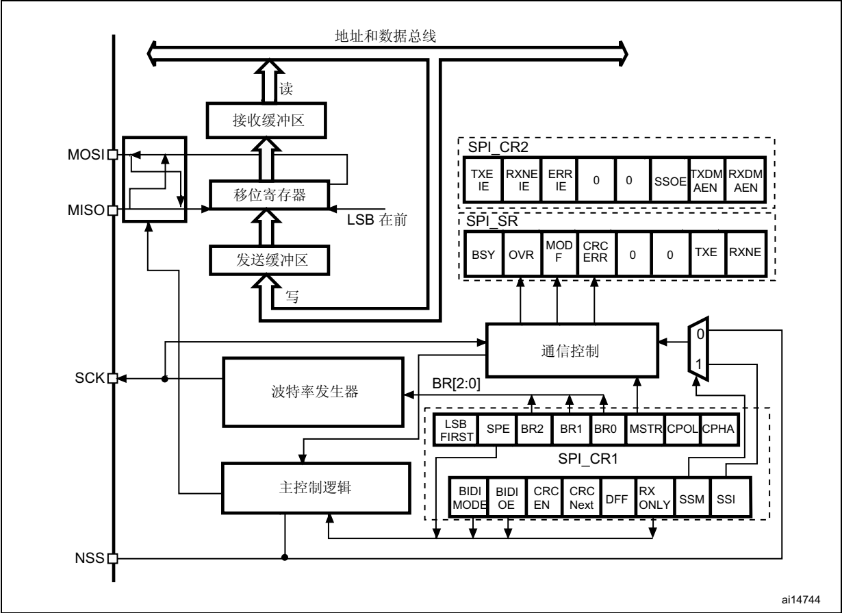
图 271. SPI 框图
