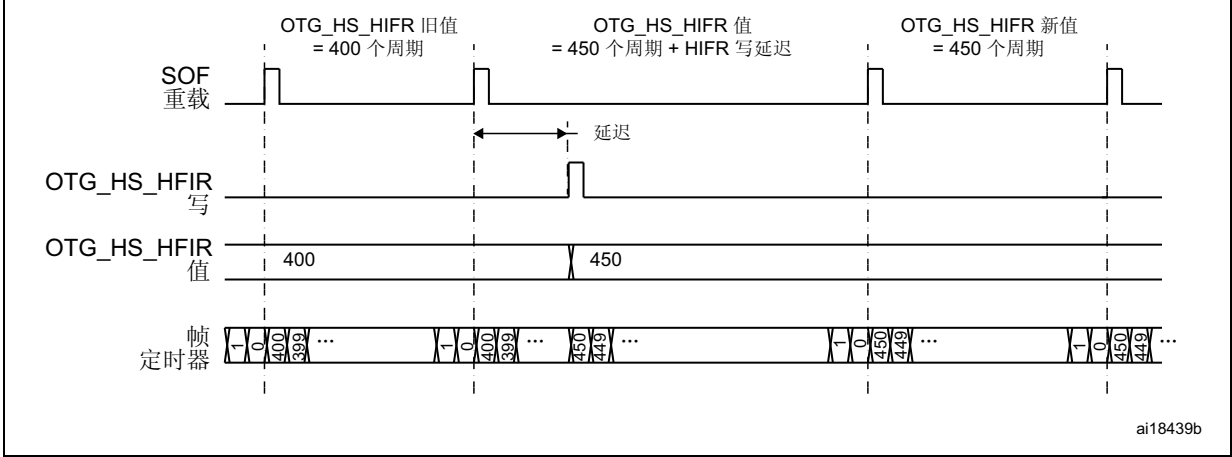
图 382. 动态更新 OTG_HS_HFIR
