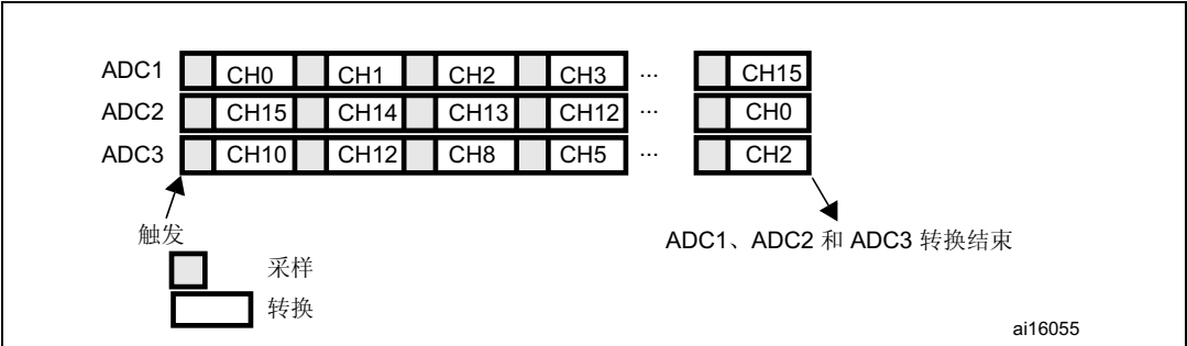
图 45. 16 通道的规则同时模式：三重 ADC 模式
