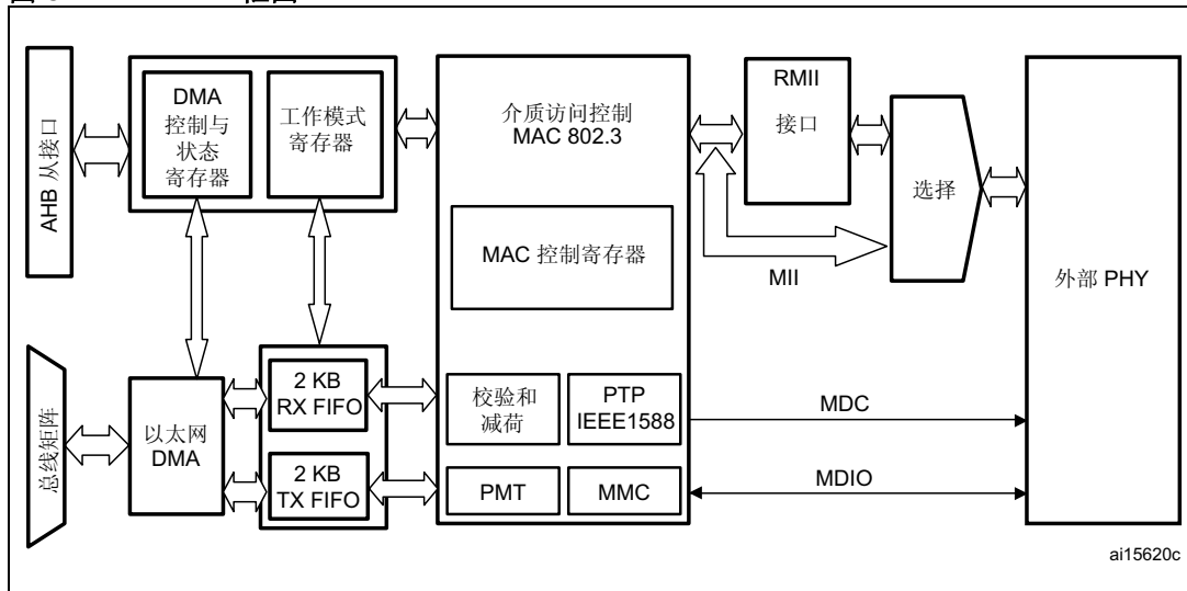
图 321. ETH 框图
