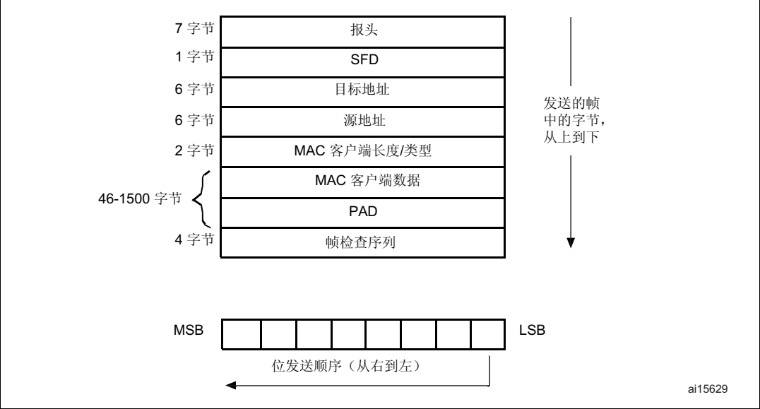
图 331. MAC 帧格式
