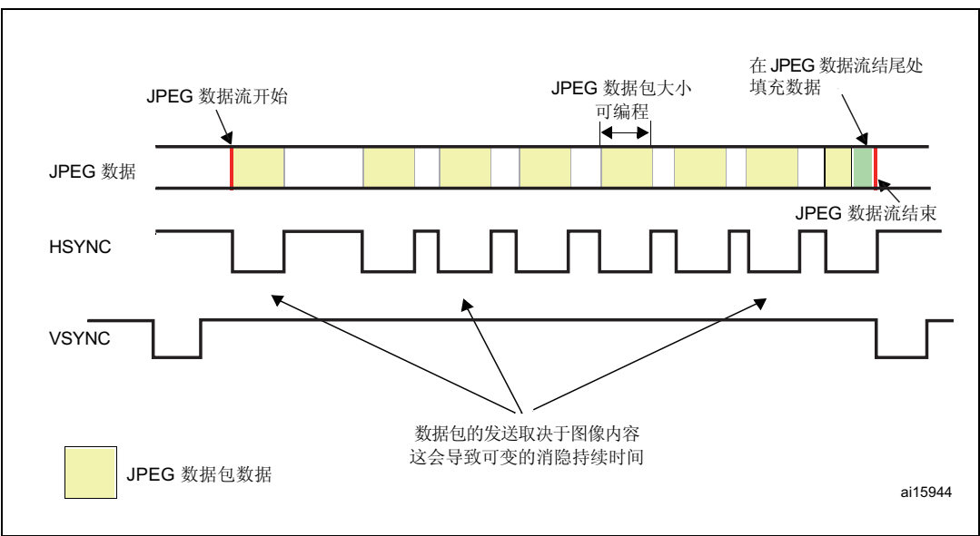
图 65. 时序图
