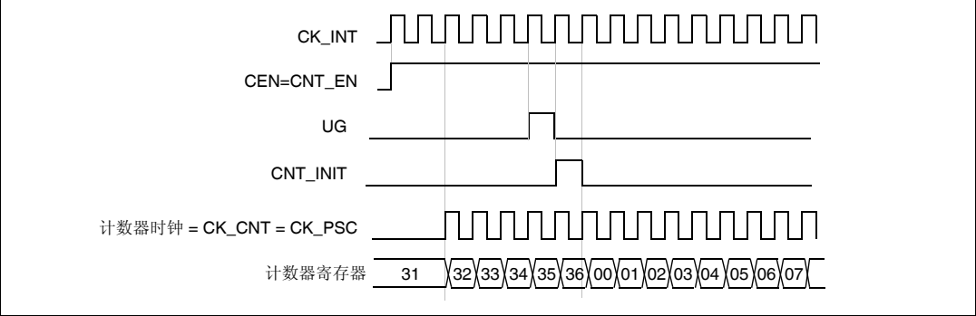
图 197. 正常模式下的控制电路，1 分频内部时钟
