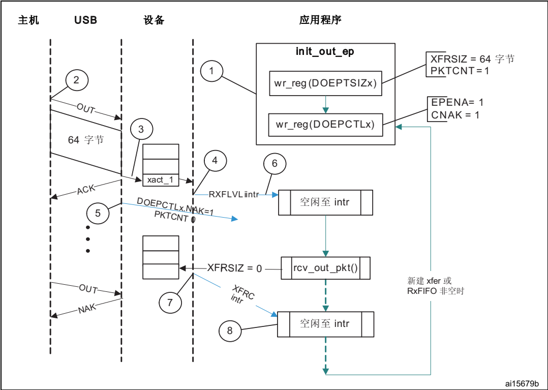
图 375. 批量 OUT 事务
