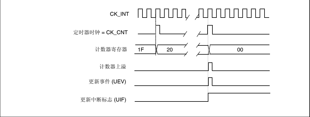
图 194. 计数器时序图，N 分频内部时钟
