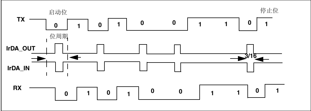
图 264. IrDA 数据调制 (3/16)——正常模式
