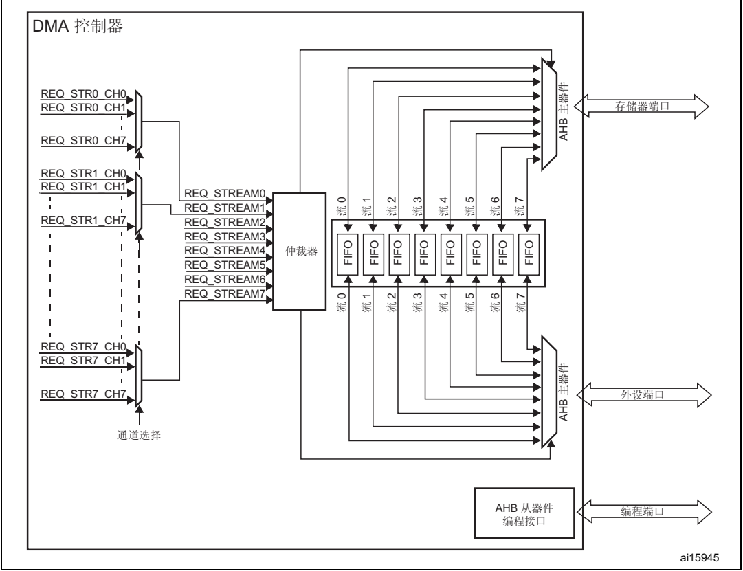
图 24. DMA 框图
