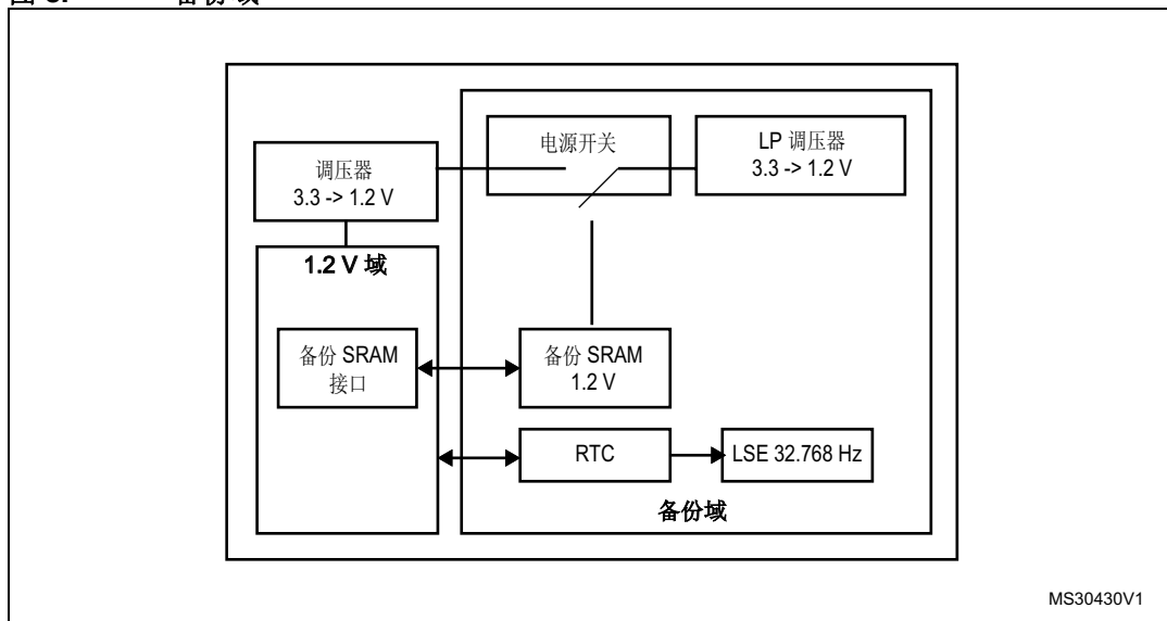
图 8. 备份域
