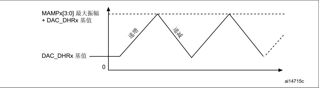
图 61. 生成三角波波形的 DAC 转换（使能软件触发）
