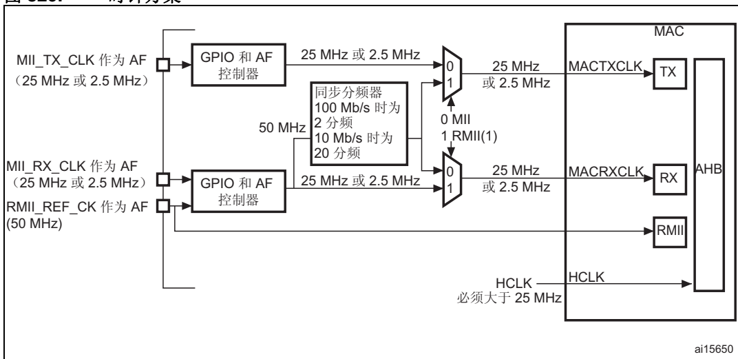
图 329. 时钟方案
