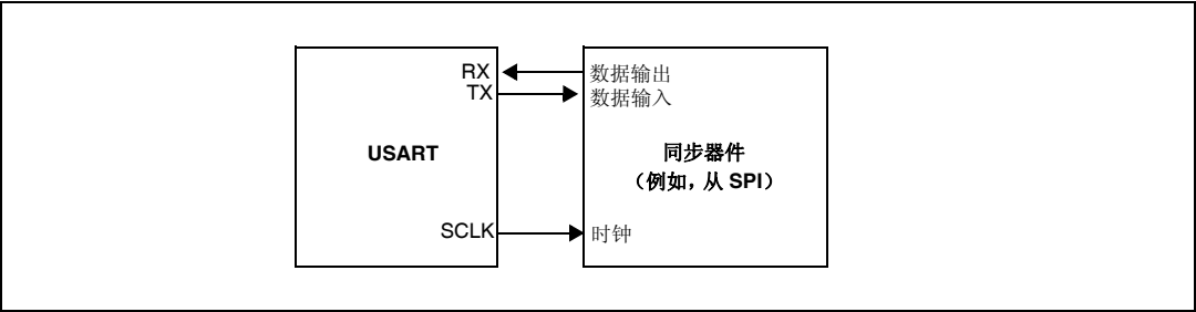
图 257. USART 同步发送示例
