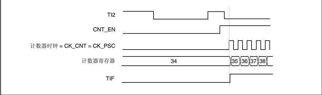
图 157. 触发模式下的控制电路
