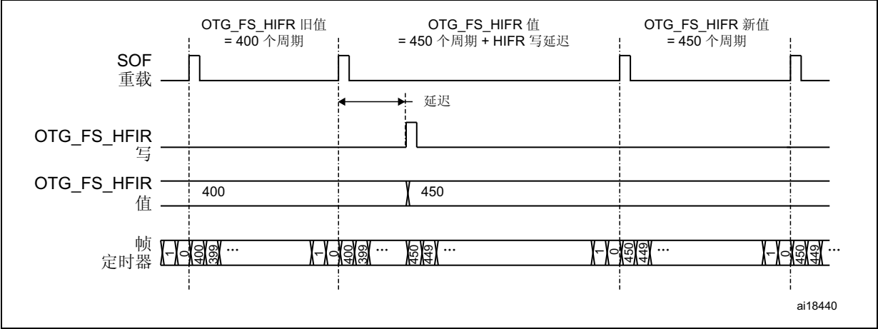
图 362. 动态更新 OTG_FS_HFIR
