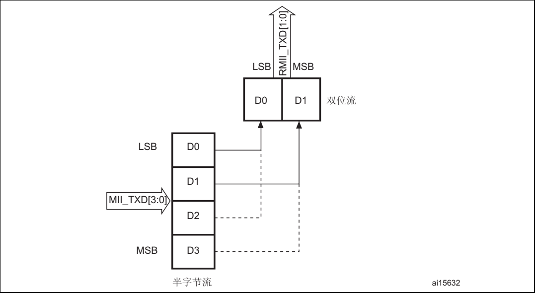
图 333. 发送位序
