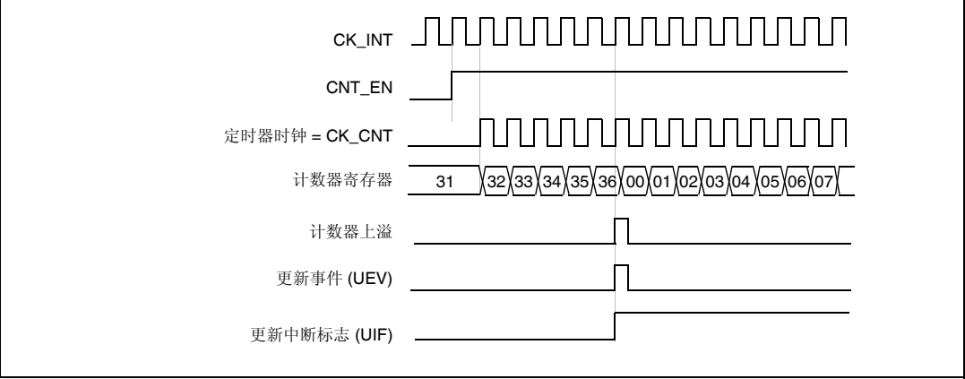
图 122. 计数器时序图，1 分频内部时钟
