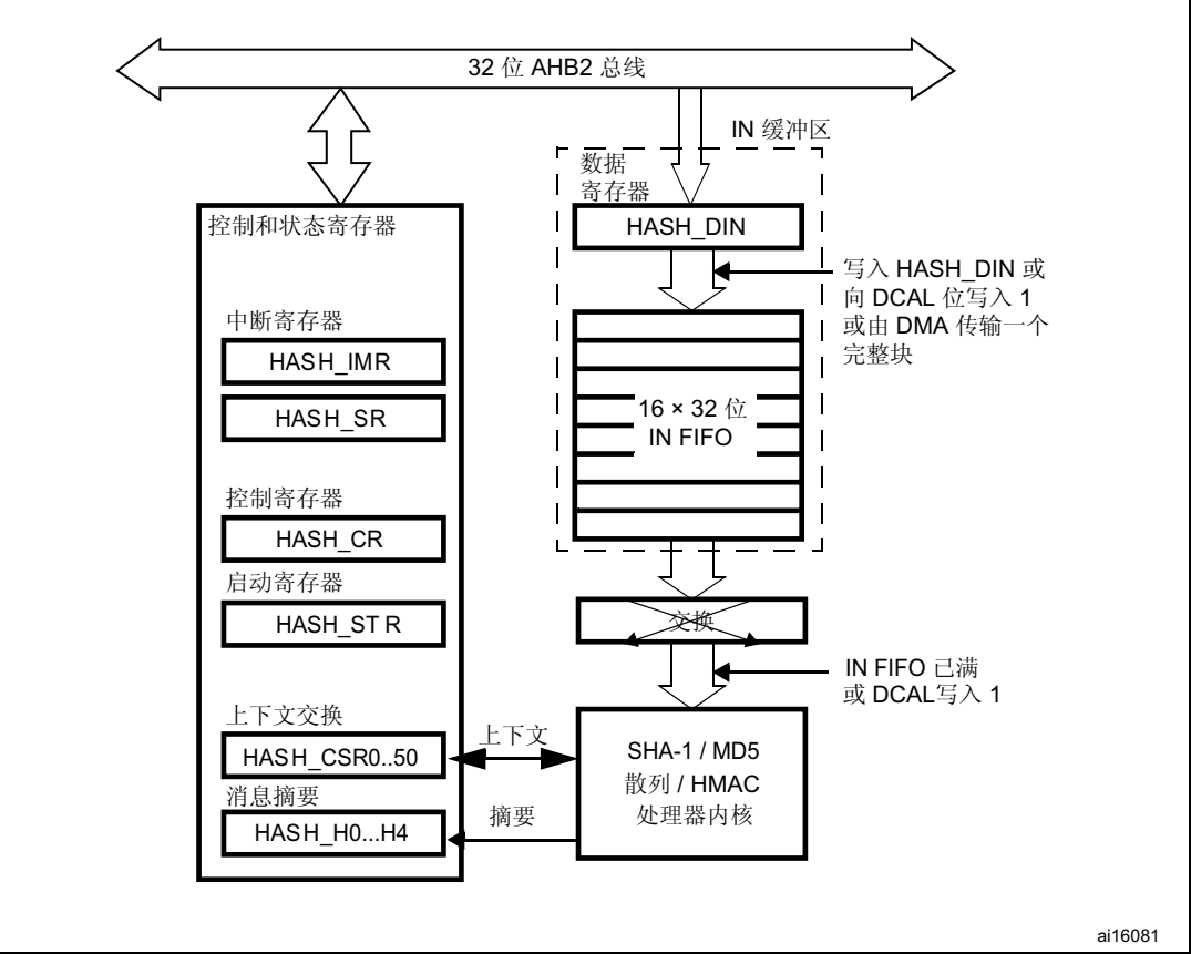
图 218. STM32F405xx/07xx 和 STM32F415xx/17xx 的框图
