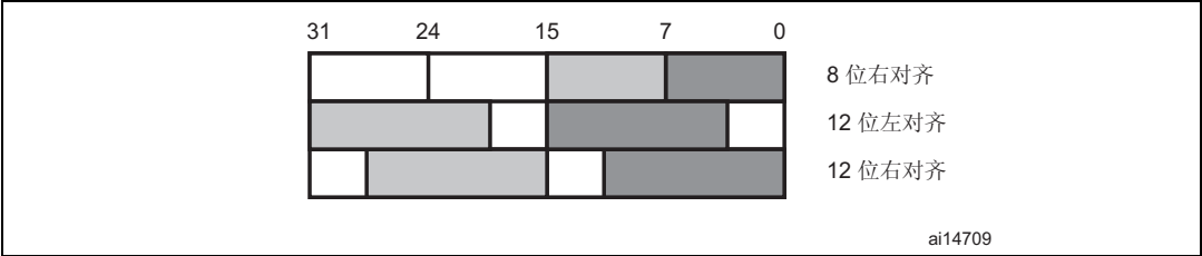
图 56. DAC 双通道模式下的数据寄存器
