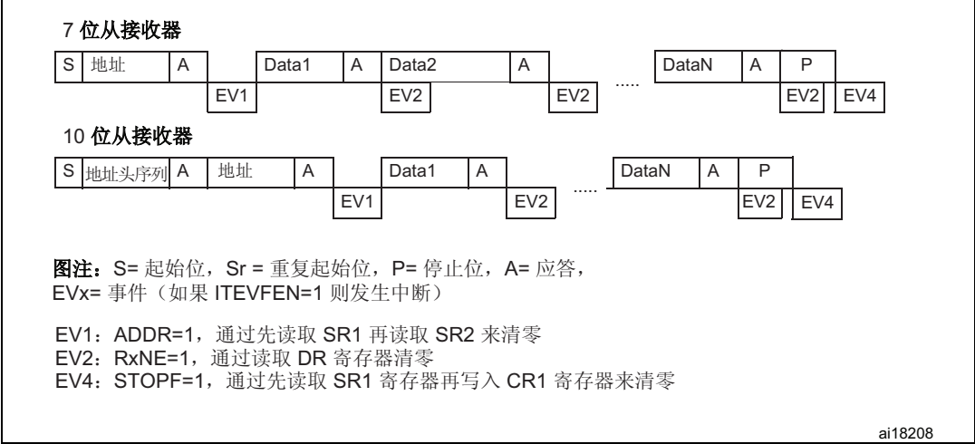
图 242. 从接收器的传输序列图
