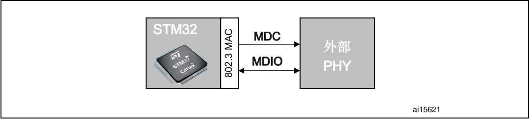
图 322. SMI 接口信号
