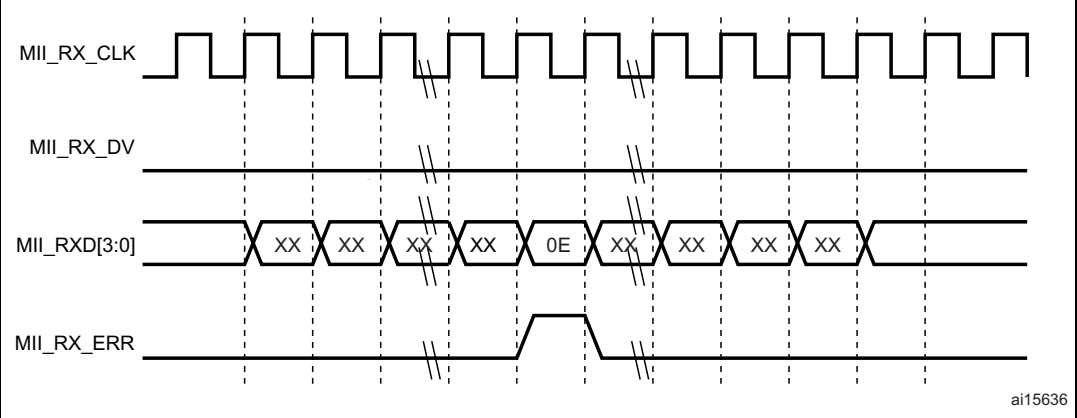
图 340. 出现假载波指示的接收
