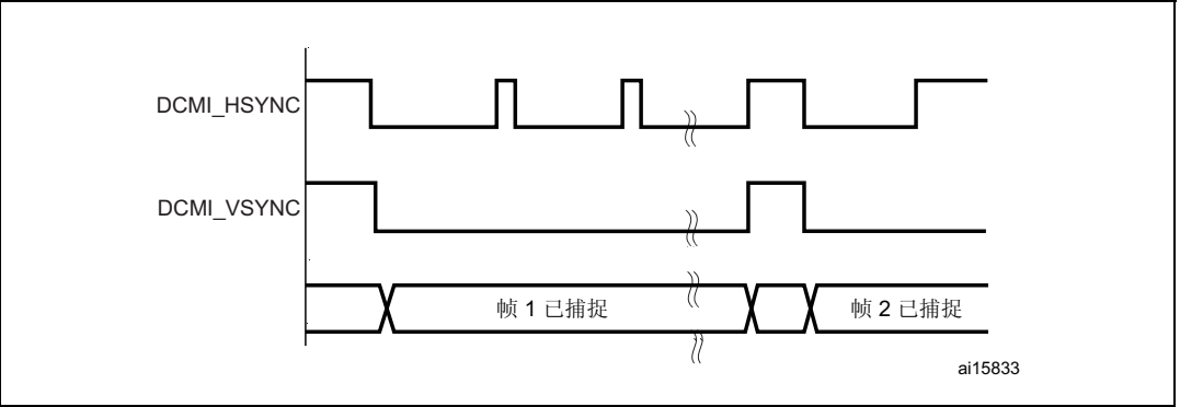
图 67. 连续采集模式下的帧捕获波形
