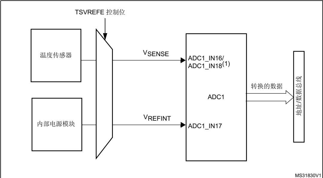
图 53. 温度传感器和 V_{REFINT} 通道框图
