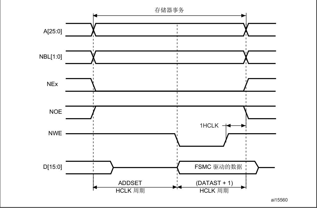
图 408. 模式 A 写入访问
