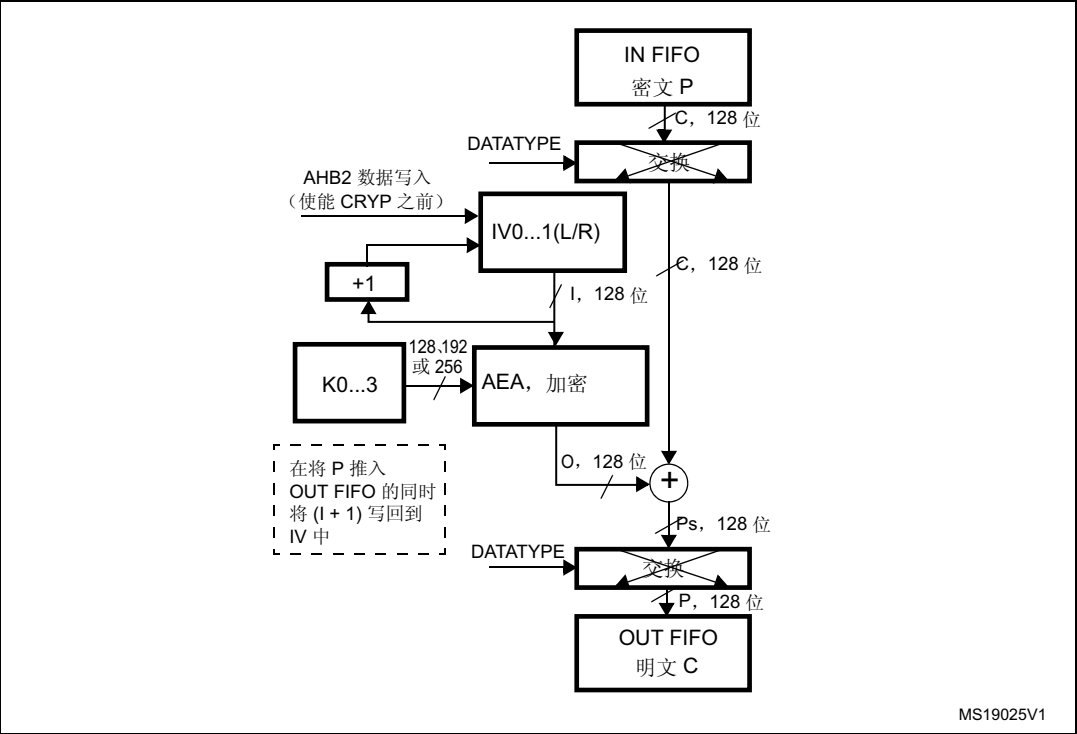
图 212. AES-CTR 模式解密
