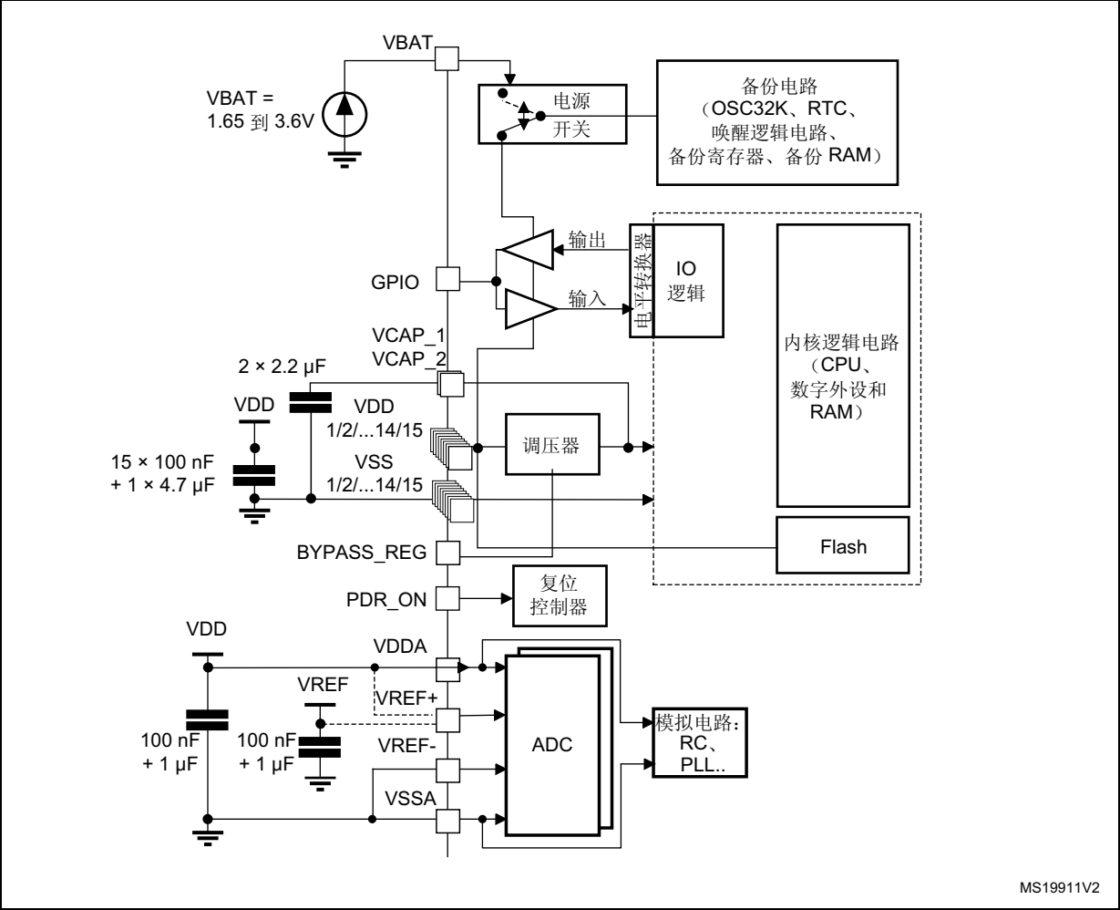
图 7. 电源概述
