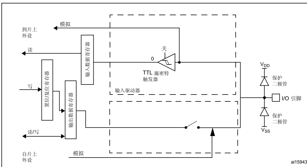
图 23. 高阻态模拟配置
