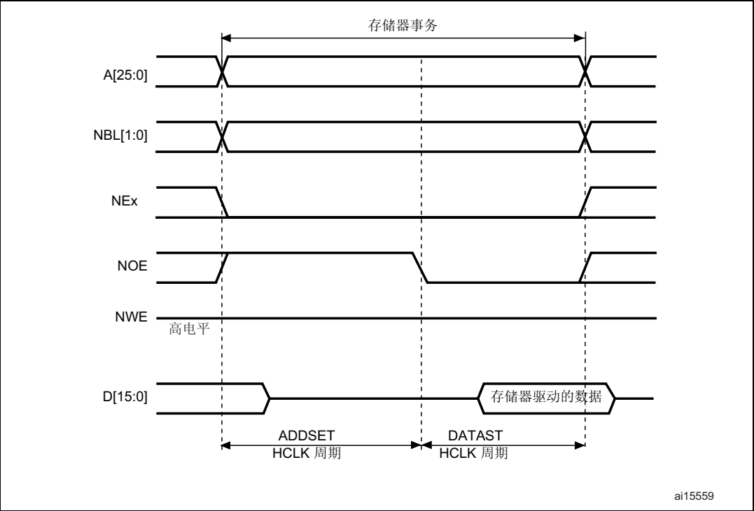
图 407. 模式 A 读取访问
