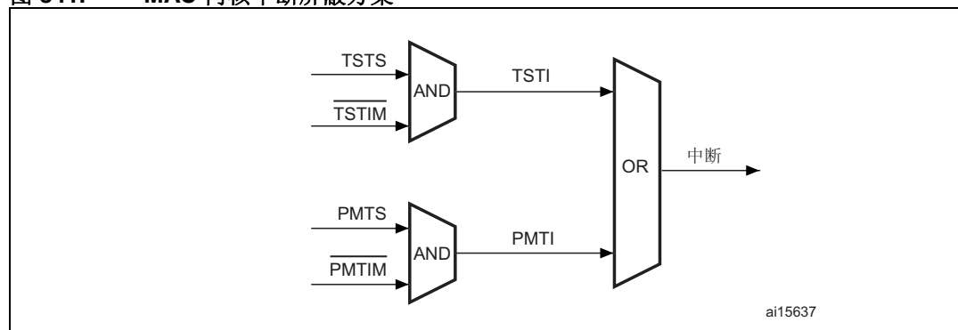
图 341. MAC 内核中断屏蔽方案
