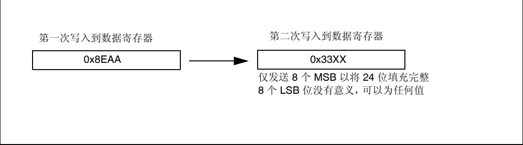
图 291. 发送 0x8EAA33
