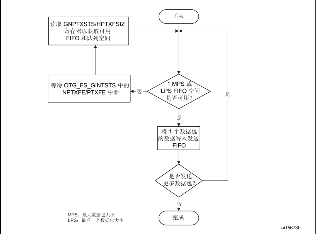
图 367. 发送 FIFO 写任务
