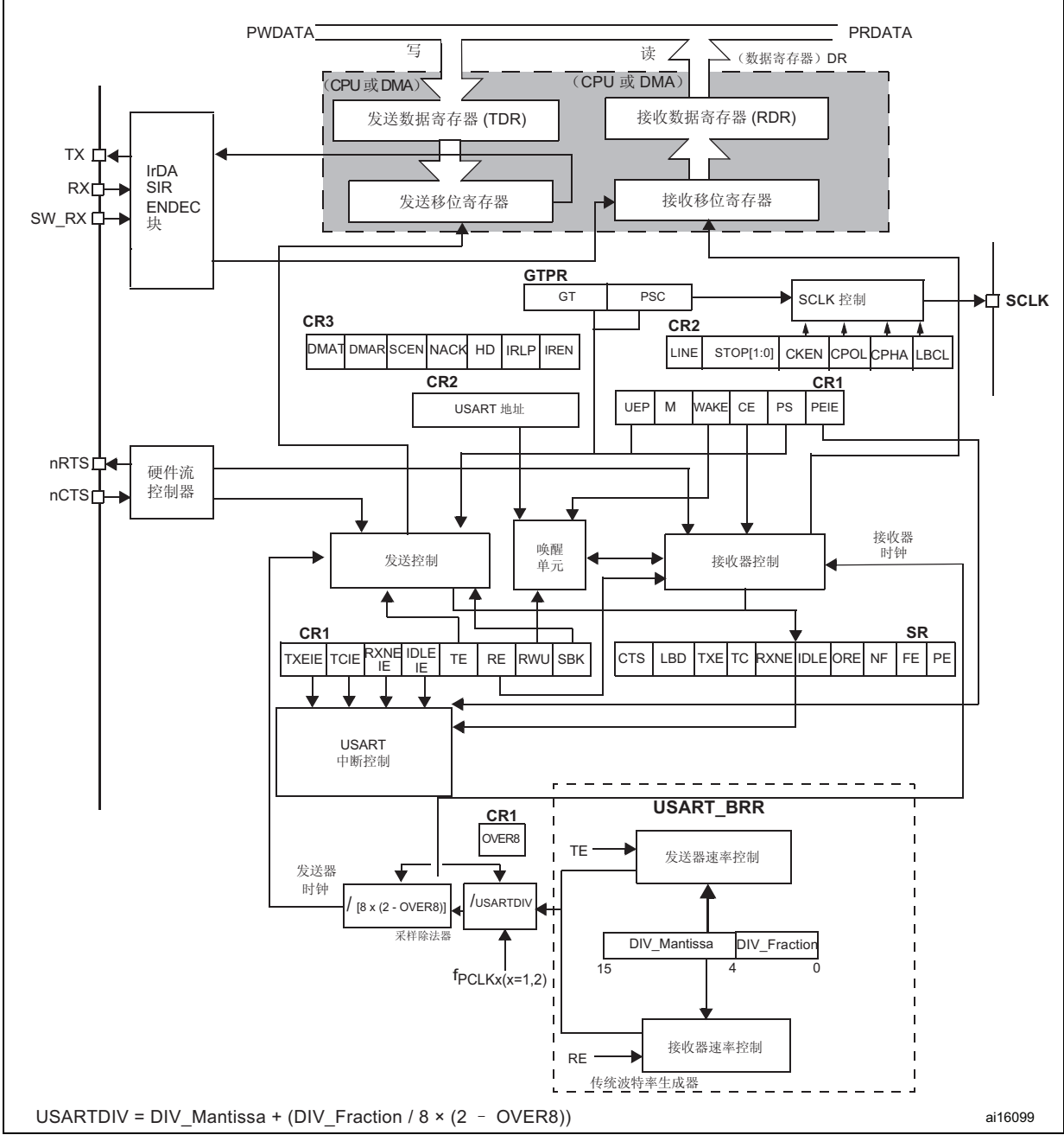
图 246. USART 框图
