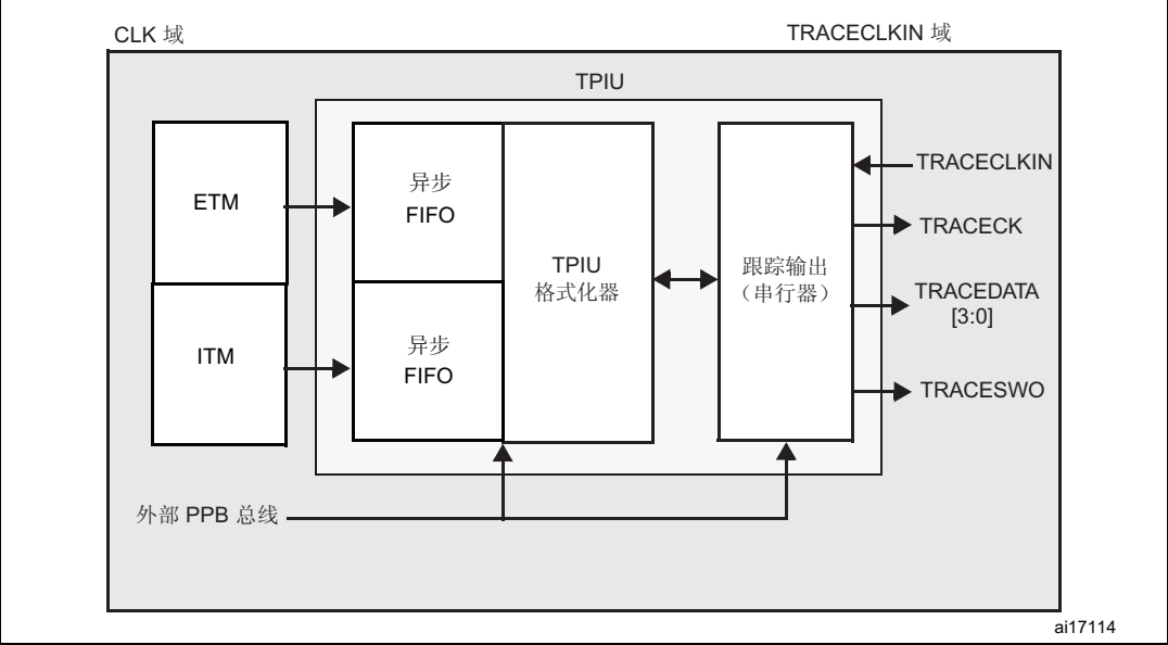
图 428. TPIU 框图
