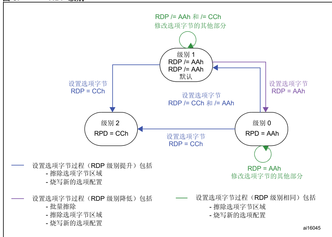
图 5. RDP 级别
