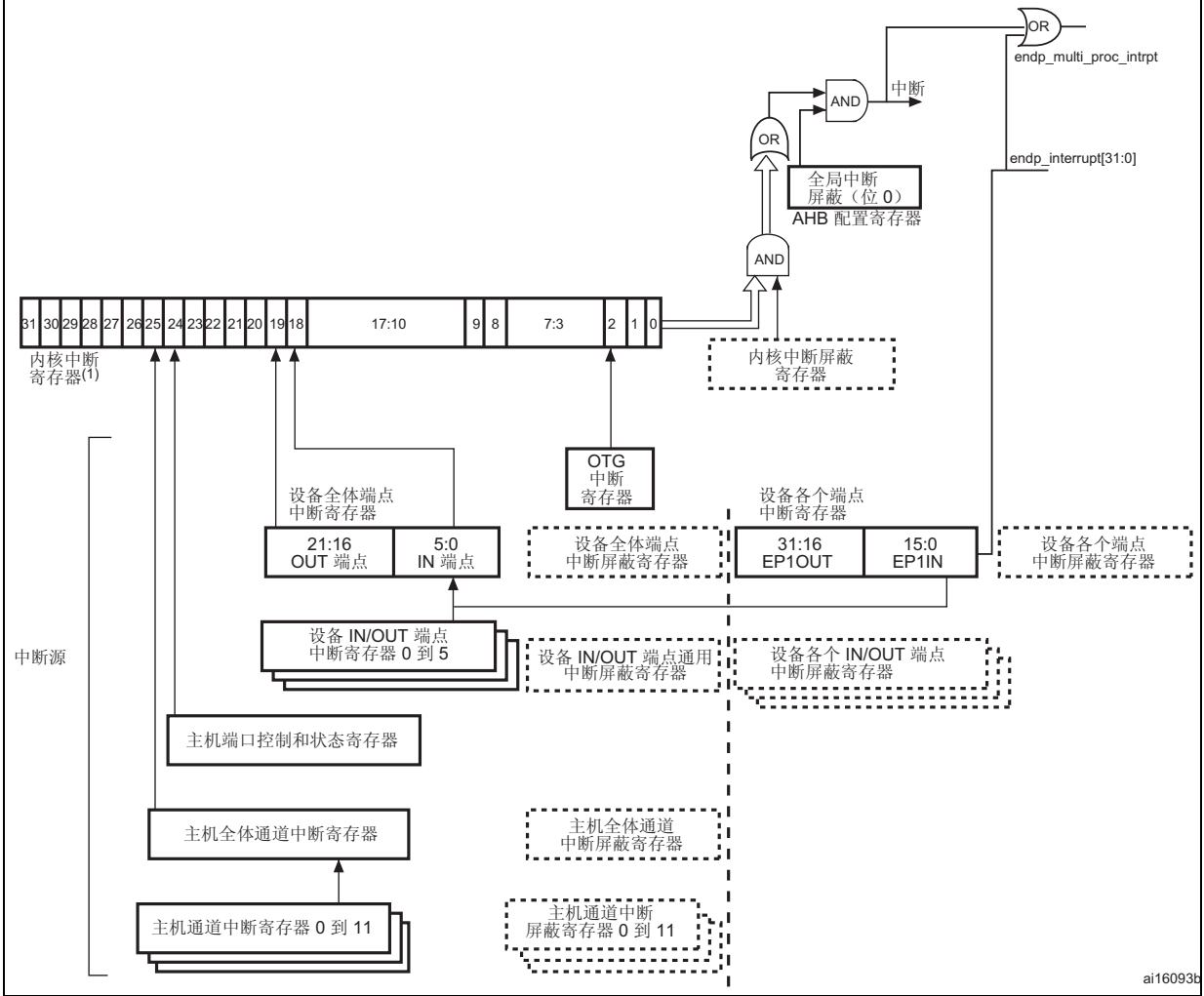
图 383. 中断层级
