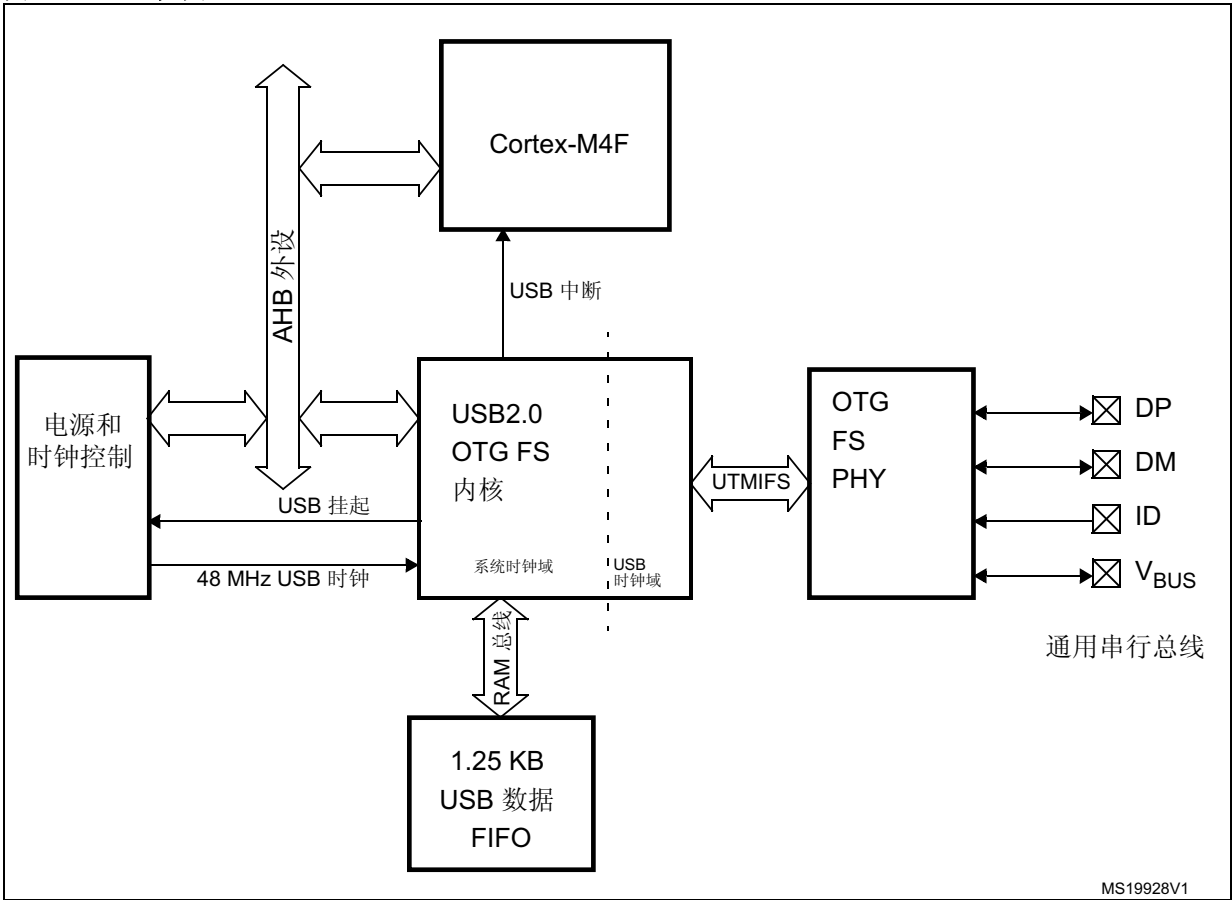
图 357. 框图
