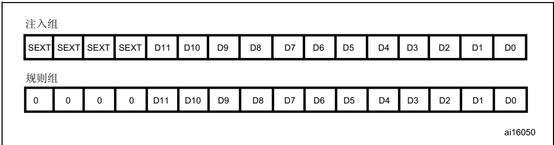
图 38. 12 位数据的右对齐
