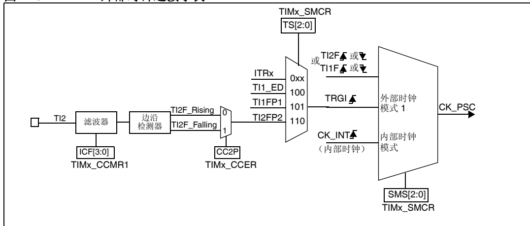
图 176. T12 外部时钟连接示例
