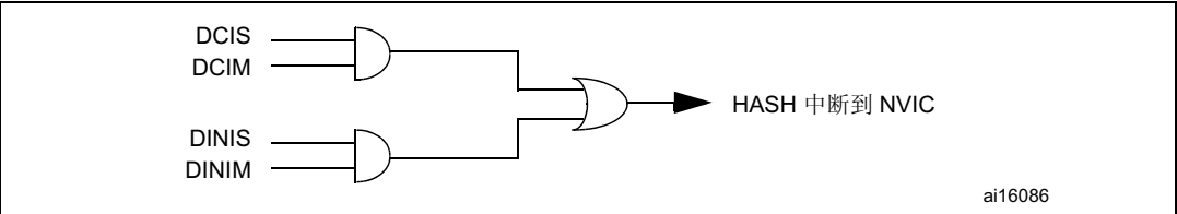
图 221. 散列中断映射图
