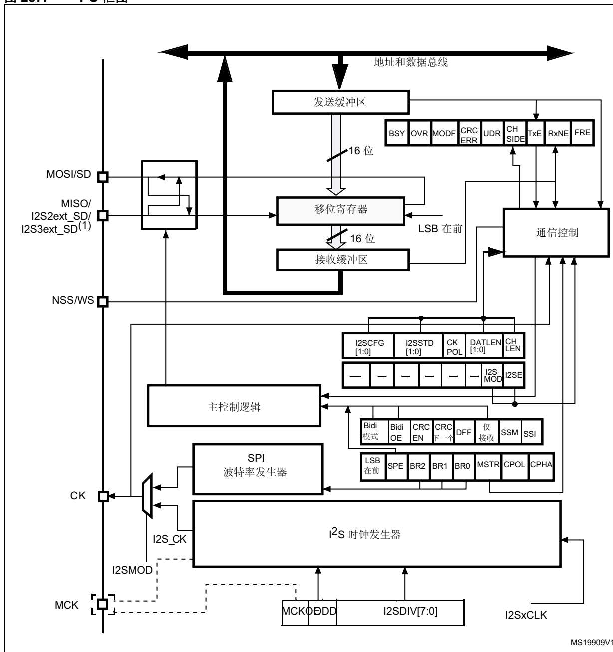
图 287. I^2S 框图
