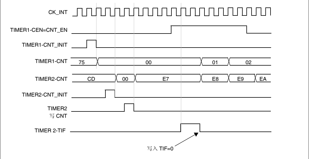
图 163. 使用定时器 1 的使能信号触发定时器 2
