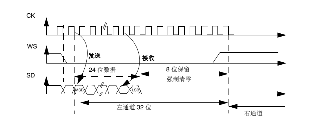
图 290. I 2 S Philips 标准波形 (24 位帧, CPOL = 0)
