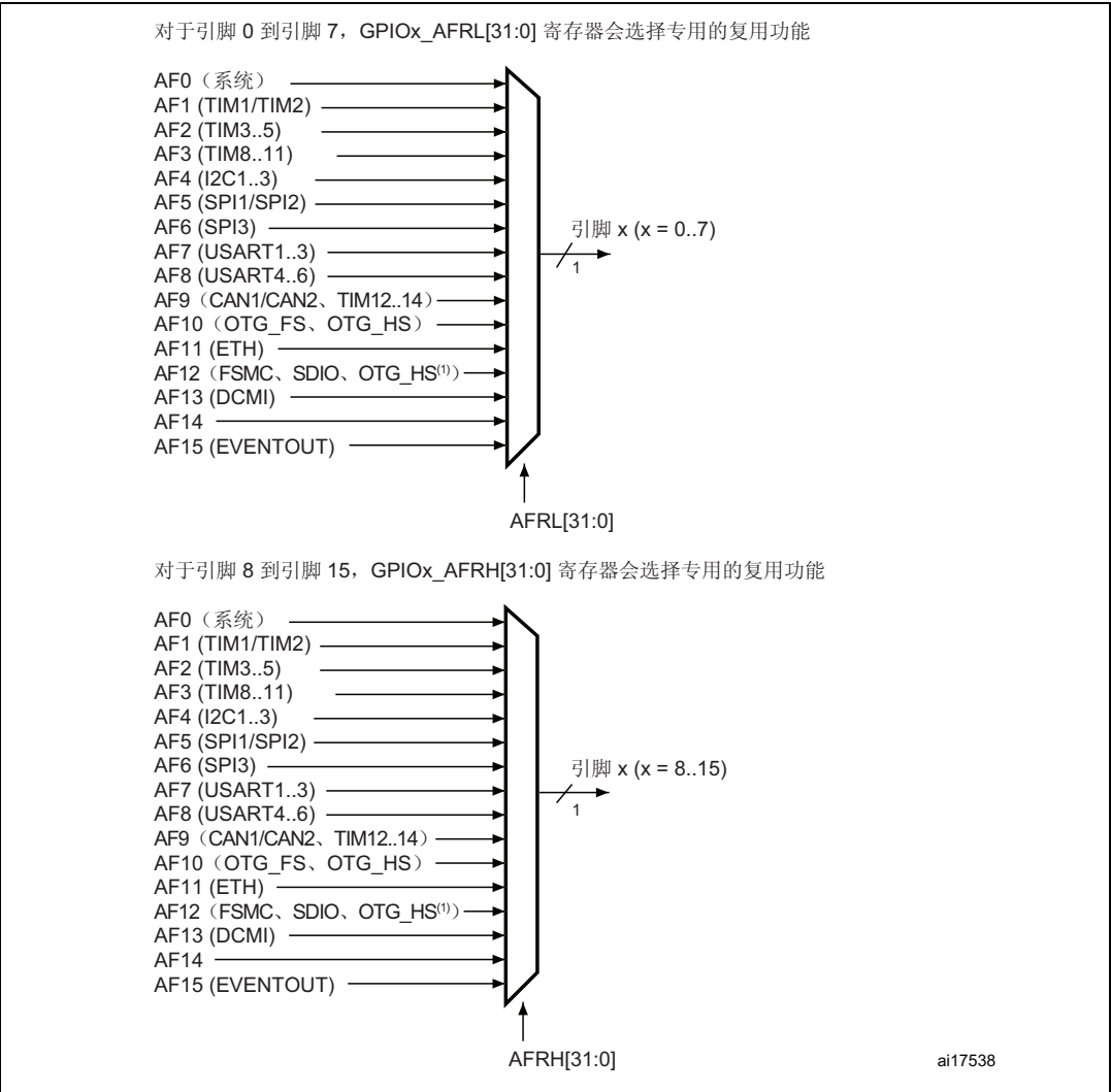
图 18. 在 STM32F405xx/07xx 和 STM32F415xx/17xx 上选择复用功能
