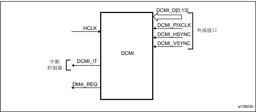
图 63. 顶级框图
