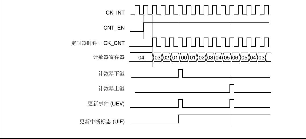
图 133. 计数器时序图，1 分频内部时钟，TIMx_ARR=0x6
