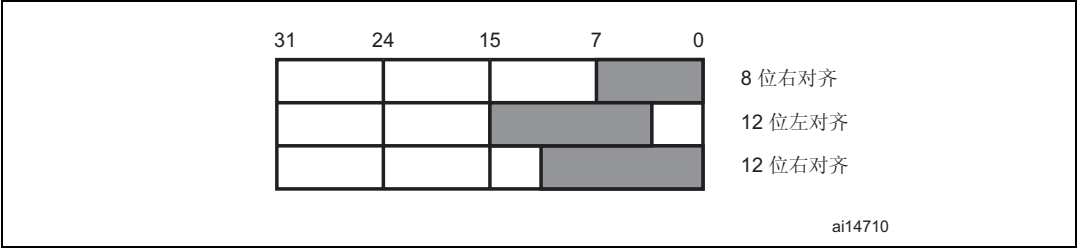
图 55. DAC 单通道模式下的数据寄存器
