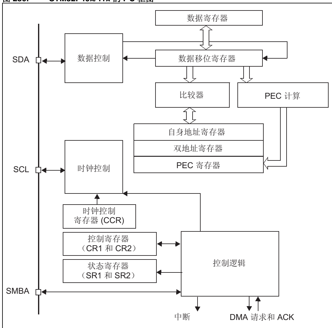
图 239. STM32F40x/41x 的 I 2 C 框图
