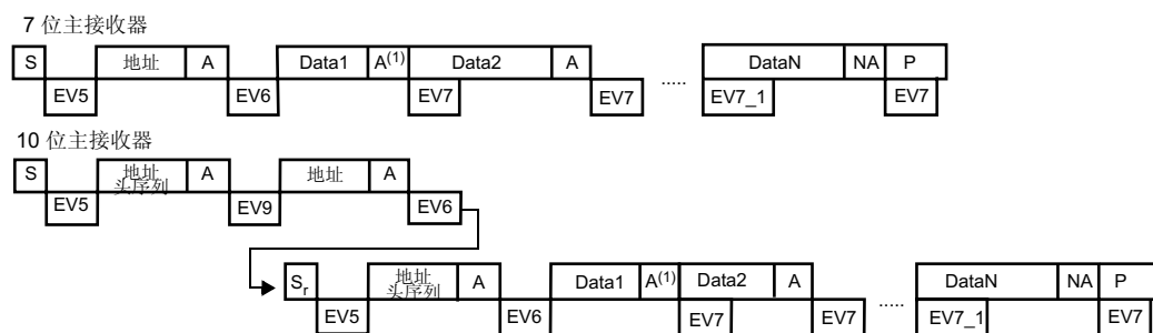
图 244. 主接收器的传输序列图
