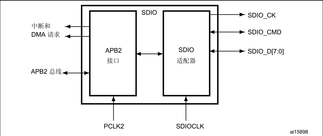
图 313. SDIO 框图
