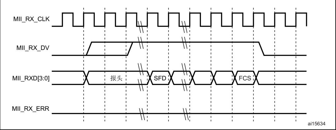
图 338. 无错误接收
