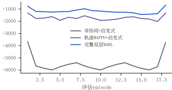
公平性
