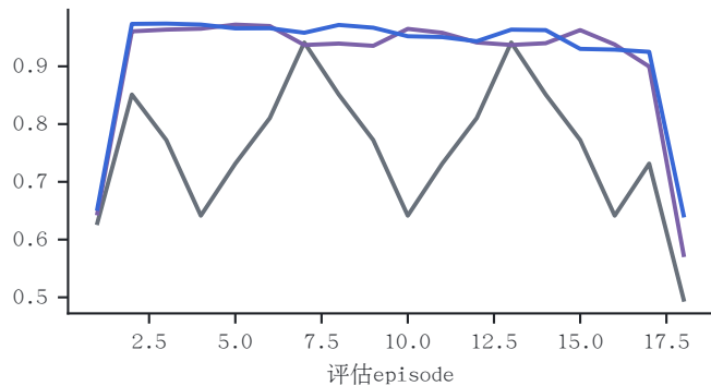
公平性
