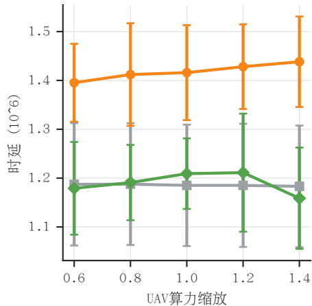
时延
