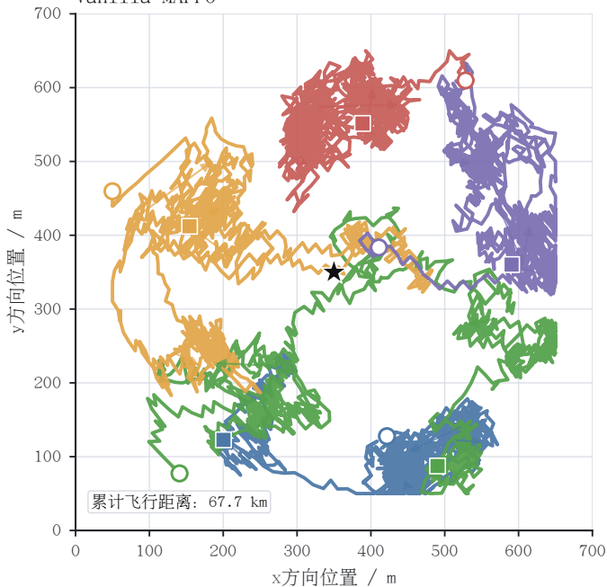
Vanilla MAPPO
