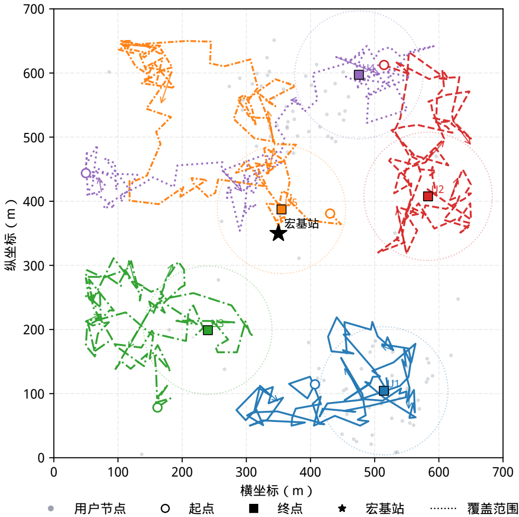
随机策略无人机二维轨迹与用户分布
