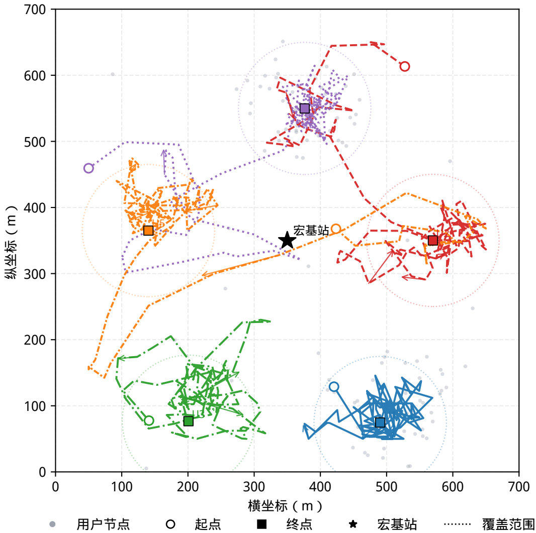
IPPO无人机二维轨迹与用户分布
