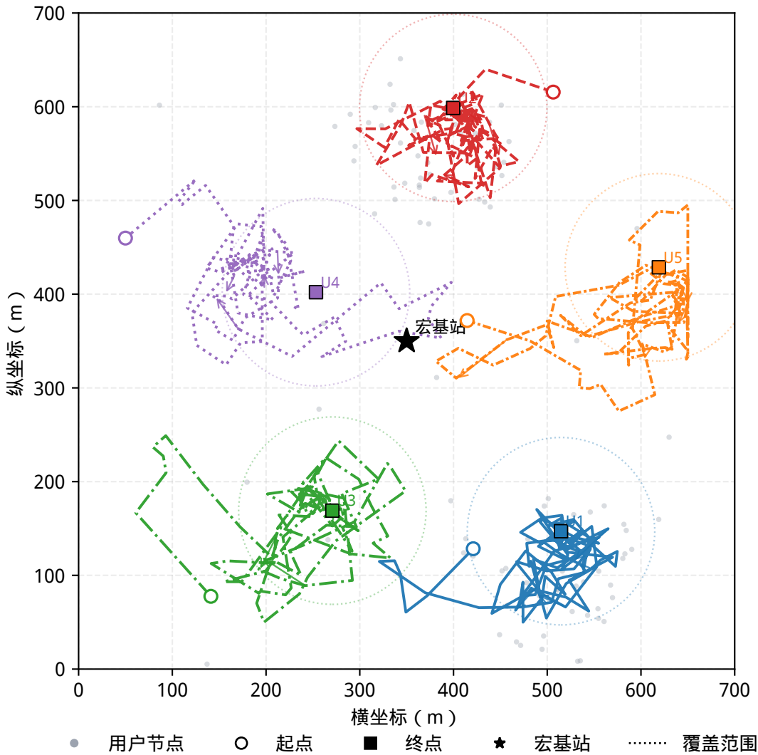
Vanilla MAPPO无人机二维轨迹与用户分布
