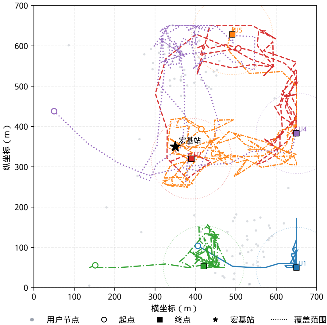
本文方法无人机二维轨迹与用户分布
