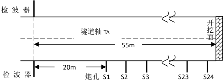
图 2 TSP 法观测系统示意图
