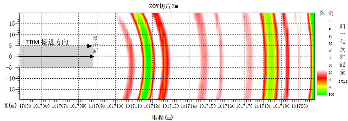
附图 2 HSP 法前方二维反演分析成果图（ZOY 切片 2m 位置-垂直切片）
