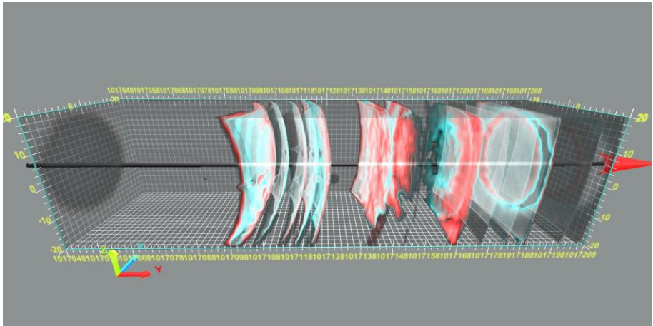
附图 3 HSP 法三维反演分析成果图（侧视图）
