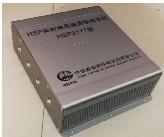
图 1 HSP217T 型地质超前预报仪
