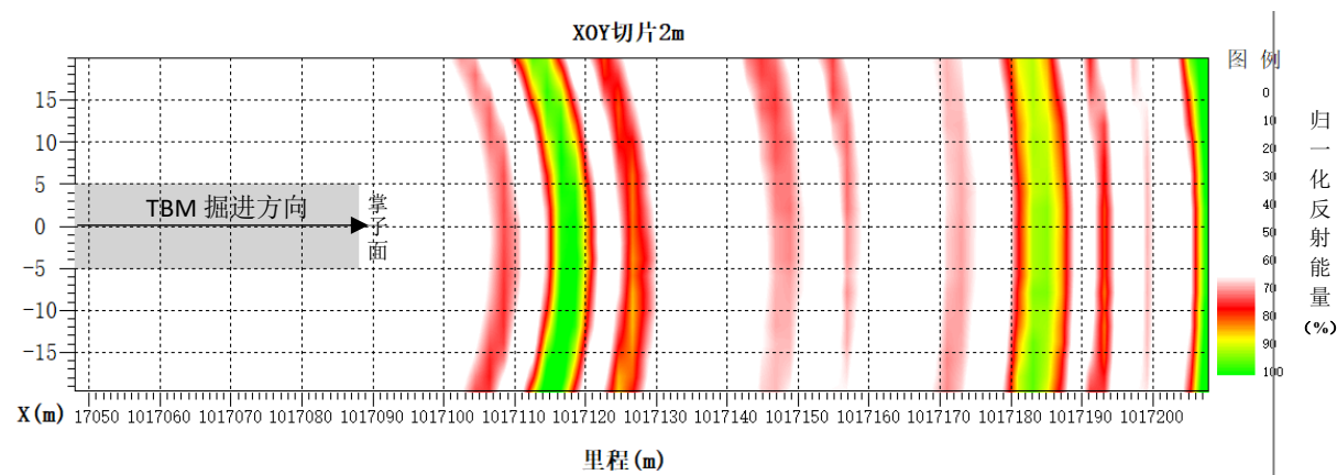
附图 1 HSP 法前方二维反演分析成果图（XOY 切片 2m 位置-水平切片）
