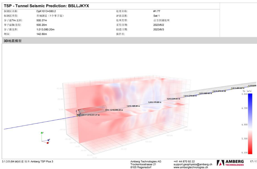
图 4 TSP 法隧道地震预报 3D 成果图
