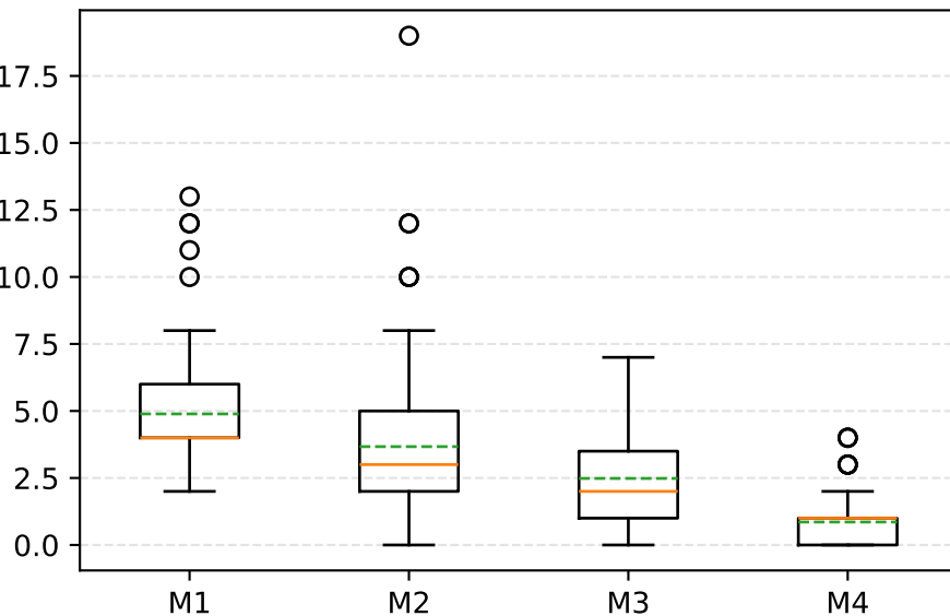
Numeric errors
